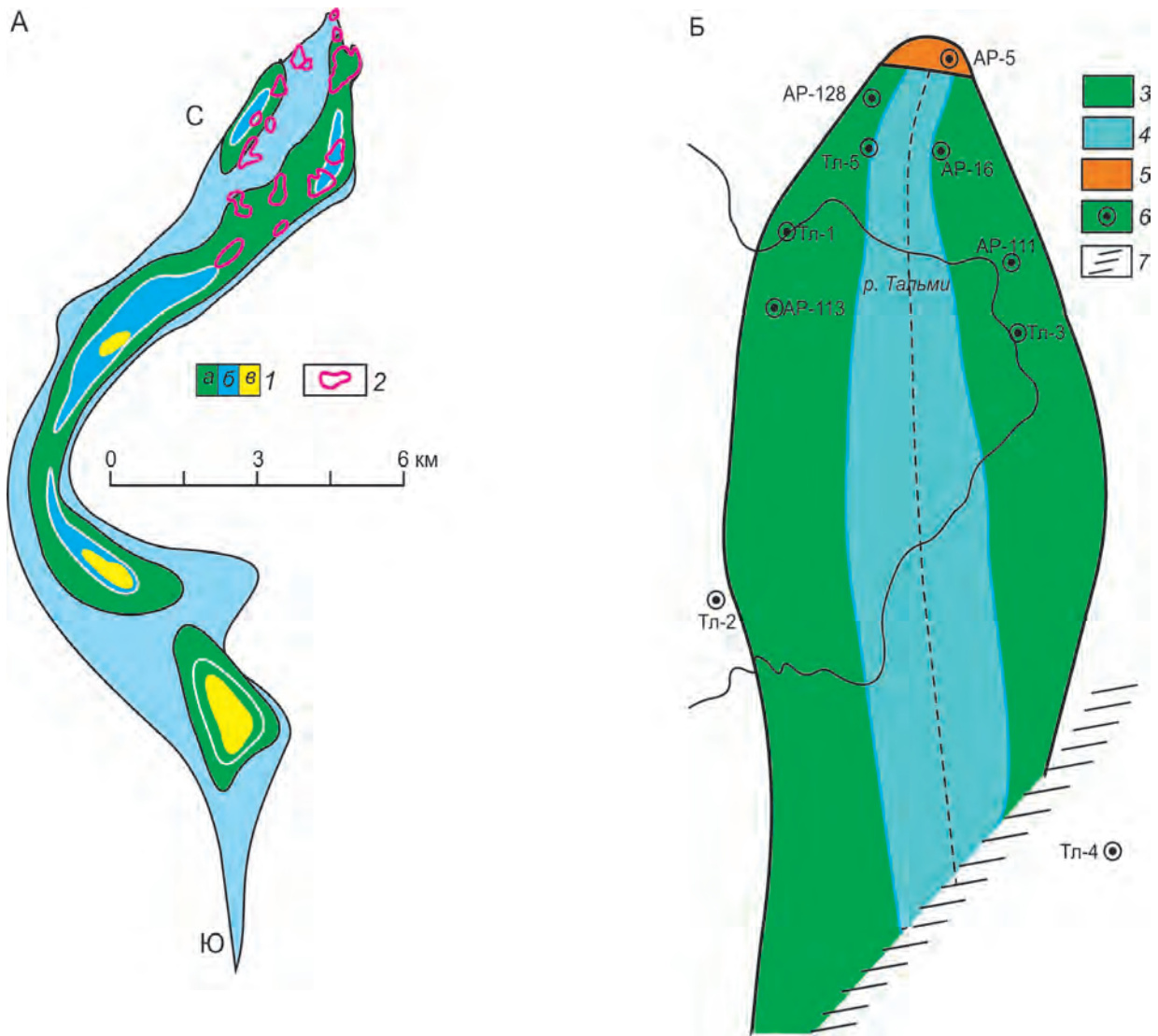
Рис. 5. Интрузия Норильск I (А) и Западная ветвь Тальминской интрузии (Б) [10]:
