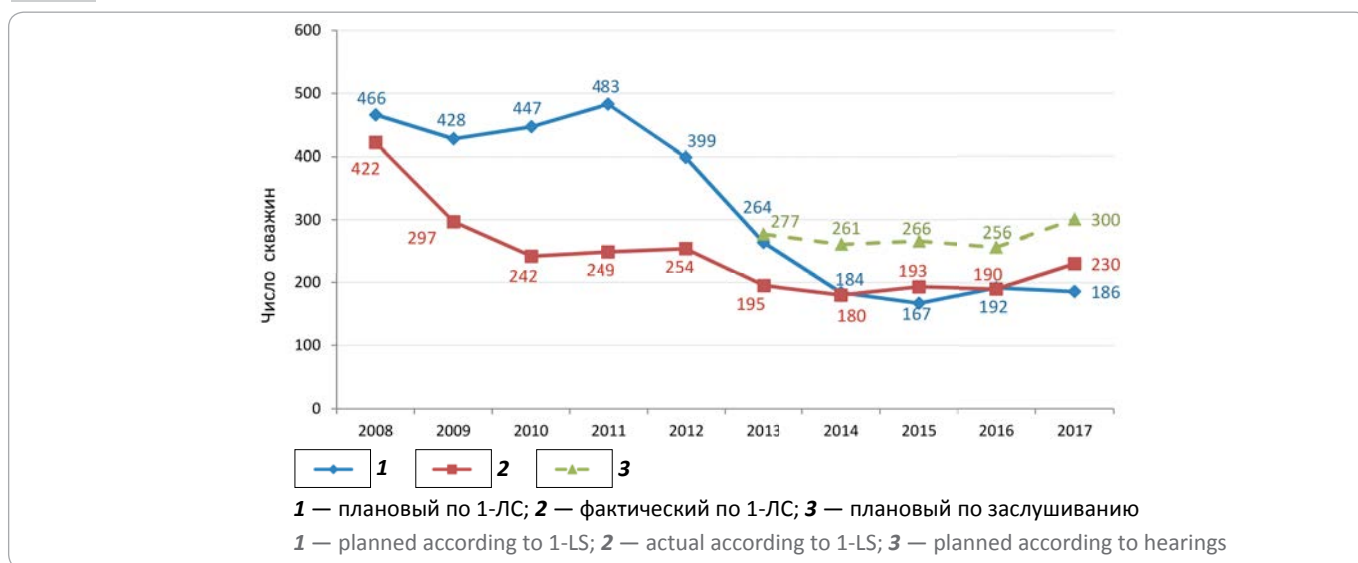
Рис. 9. Выполнение объемов поискового и оценочного бурения по РФ за 2008–2017 гг. по данным 1-ЛС Fig. 9. Amount of prospecting and appraisal drilling in Russia during 2008–2017 according to 1-LS form
