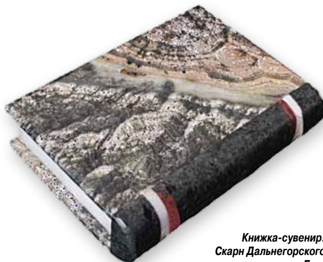
Геденбергит-волластонитовый скарн с полостью, выполненной датолитом и апофиллитом. Дальнегорск, месторождение Бор.
