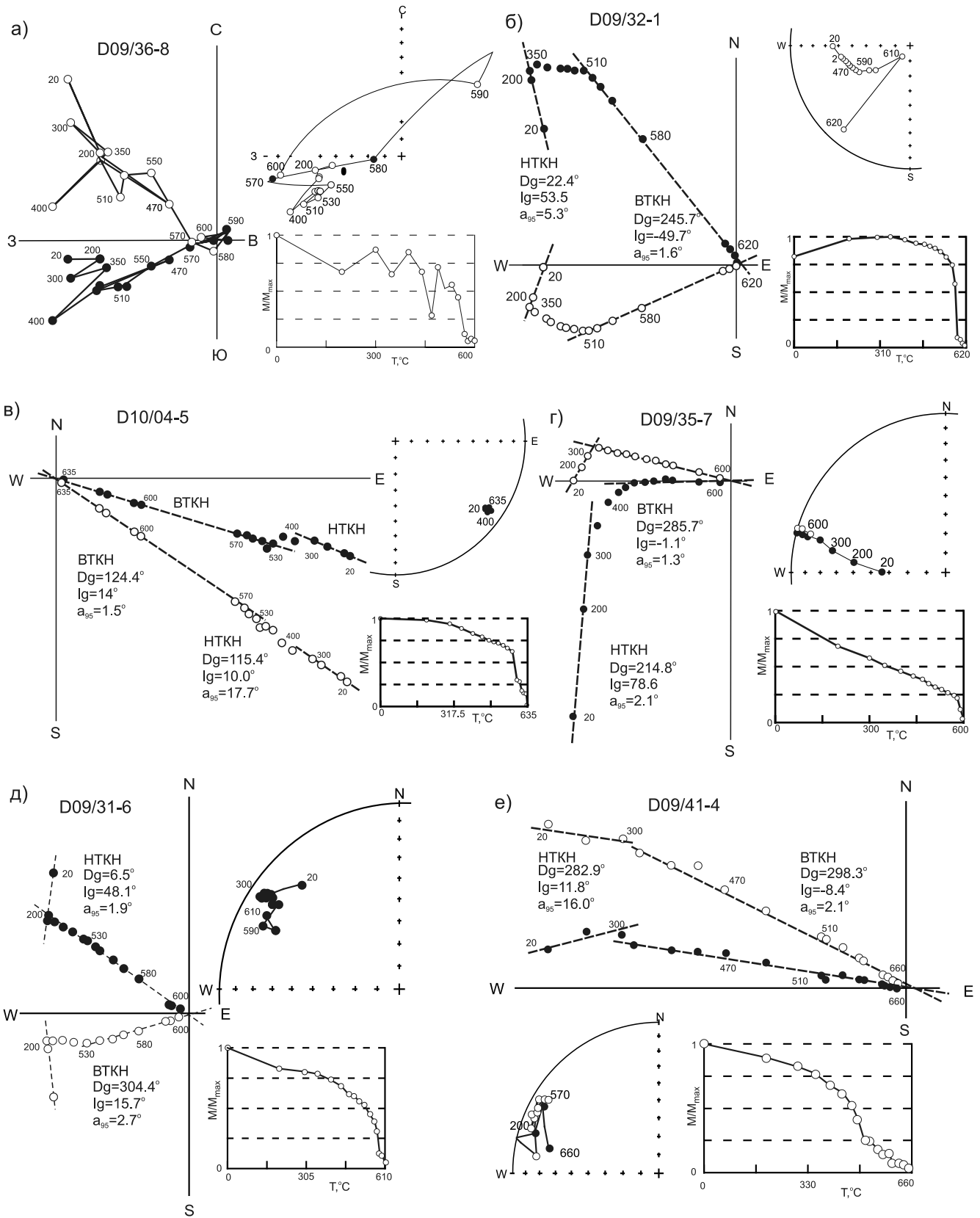
Рис. 7. Примеры ступенчатого терморазмагничивания NRM пород Киселевского блока на диаграммах Зийдерверльда [66]. Диаграммы: а, в, г – базальтов; б, д, е – алевролитов. Залитые знаки – проекция на горизонтальную плоскость, полые – на вертикальную. Числа у знаков – температура магнитной чистки в °С.
