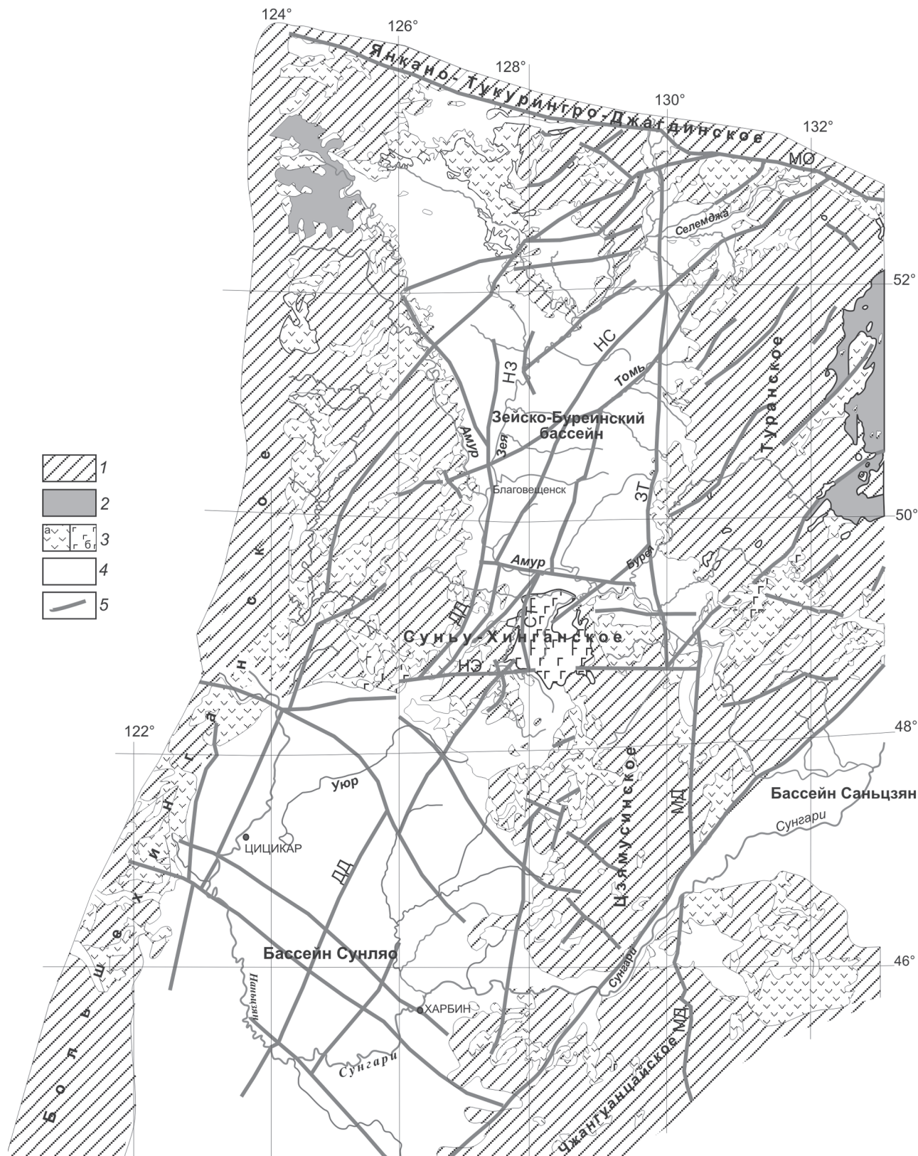
Рис. 1. Схема морфоструктурного районирования Восточно-Азиатского рифтогенного пояса.
