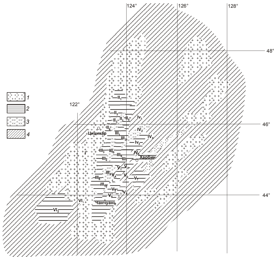
Рис. 2. Тектоническое районирование бассейна Сунляо [2].
