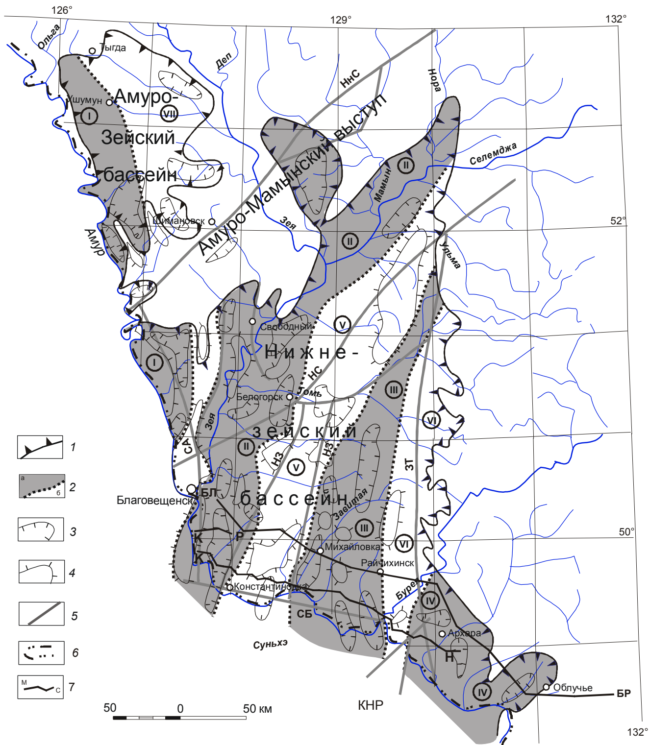
Рис. 3. Тектоническая схема Зейско-Буреинского бассейна (по [6, 18, 33]).
