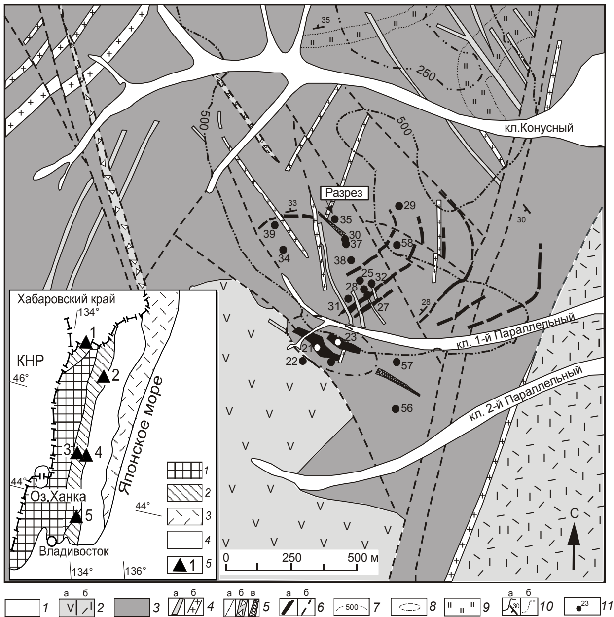
Рис. 1. Схематическая геологическая карта месторождения Кордонного (по материалам П.В. Кораблинова и др., 1985 г., с добавлениями А.В. Гурикова и С.И. Садкина).
