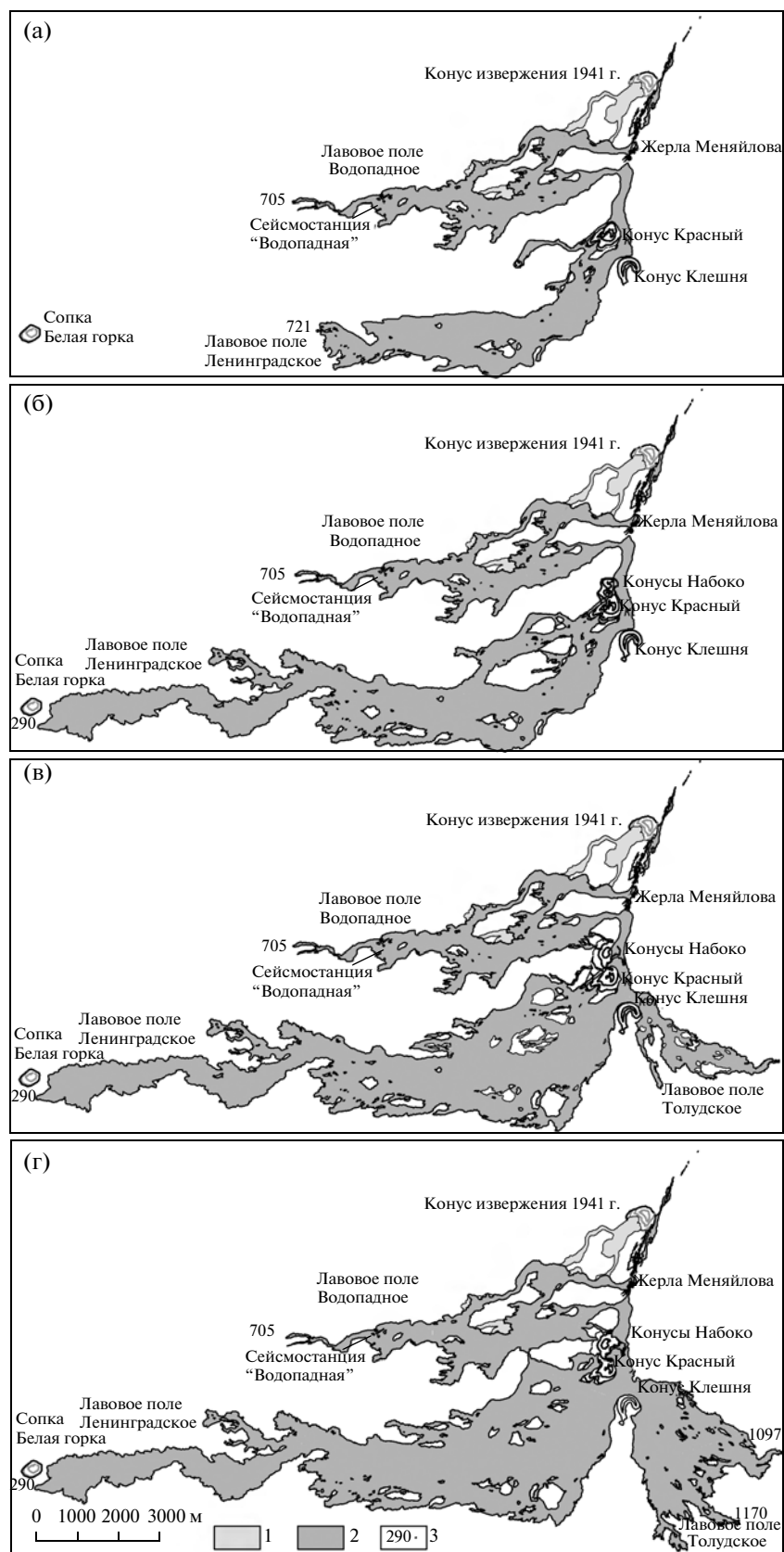
Рис. 3. Последовательность развития лавовых полей ТТИ. а – 29.11.2012; б – 13.12.2012; в – 06.03.2013; г – 05.06.2013.
