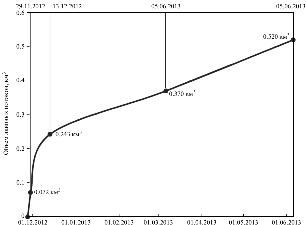
Рис. 2. График изменения объемов лавовых потоков за первые полгода ТТИ 2012–2013 гг.
