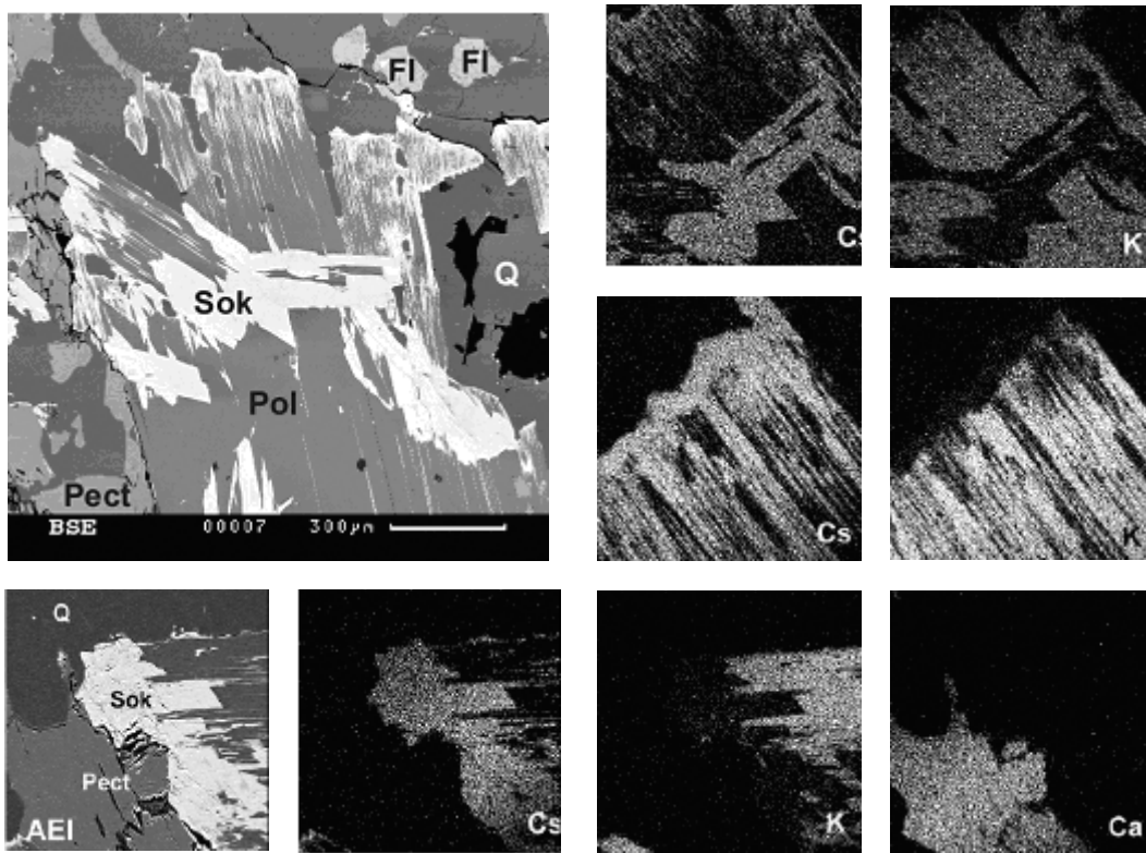
Рис. 4. Странствие соколоваита (Sok) с полилитионитом (Pol) в кварц (Q) – пектолитовом (Pect) агрегате. Обзорное изображение полированного шлифа в отраженных электронах (BSE) и фрагментов в характеристическом рентгеновском излучении указанных элементов
