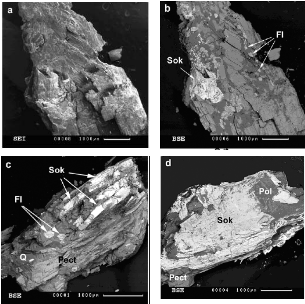
Рис. 3. Характер выделений соколоваита в полиминеральном существенно пектолитовом агрегате. Sok – соколоваит, Pect – пектолит, Q – кварц, Pol – поллитоинит, Fl – стронцийсодержащий флюорит. РЭМ-фото. a, b – гнездобразное выделение соколоваита в пектолит-кварцевом агрегате; c – лейсты соколоваита в кварце с пектолитом. d – пластинчатые зерна соколоваита в сростании с поллитоинитом.
