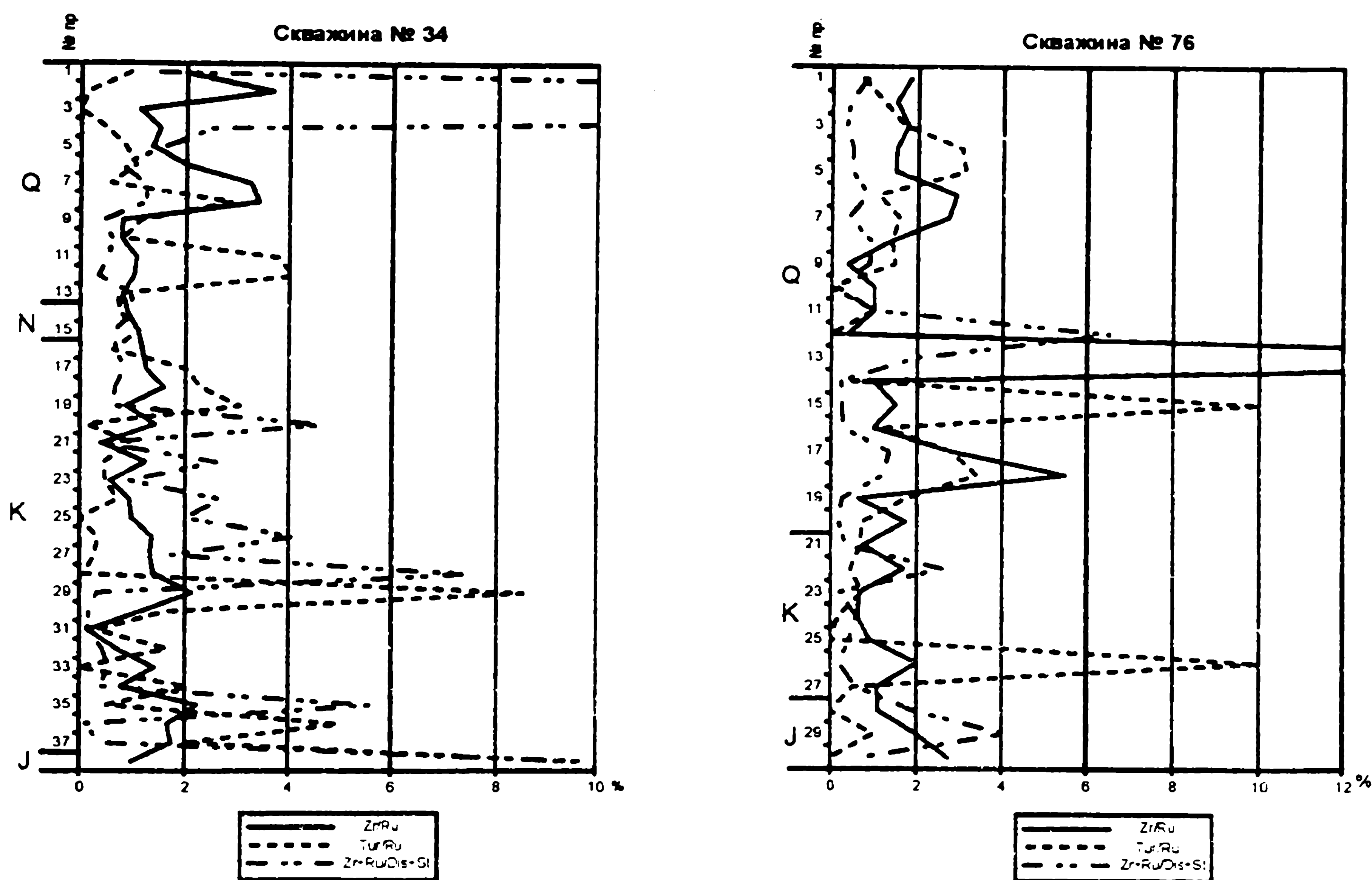
Рис. 3. Графики значений минералогических коэффициентов по скважинам
