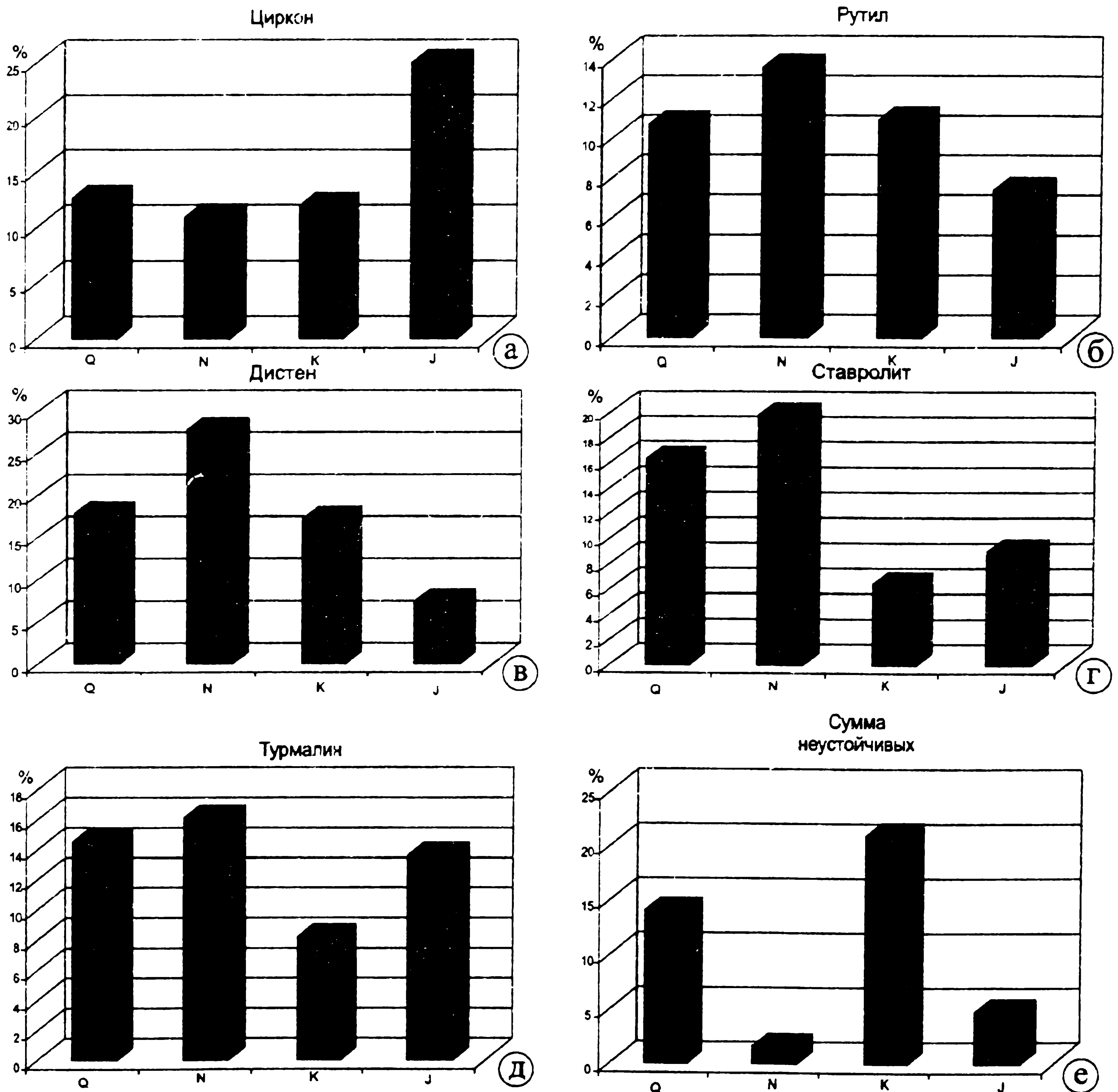
Рис. 1. Диаграммы распределения акцессорных минералов: а) циркона; б) рутила; в) дистена; г) ставролита; д) турмалина; е) суммы неустойчивых (продолжение рисунка на следующей стр.)
