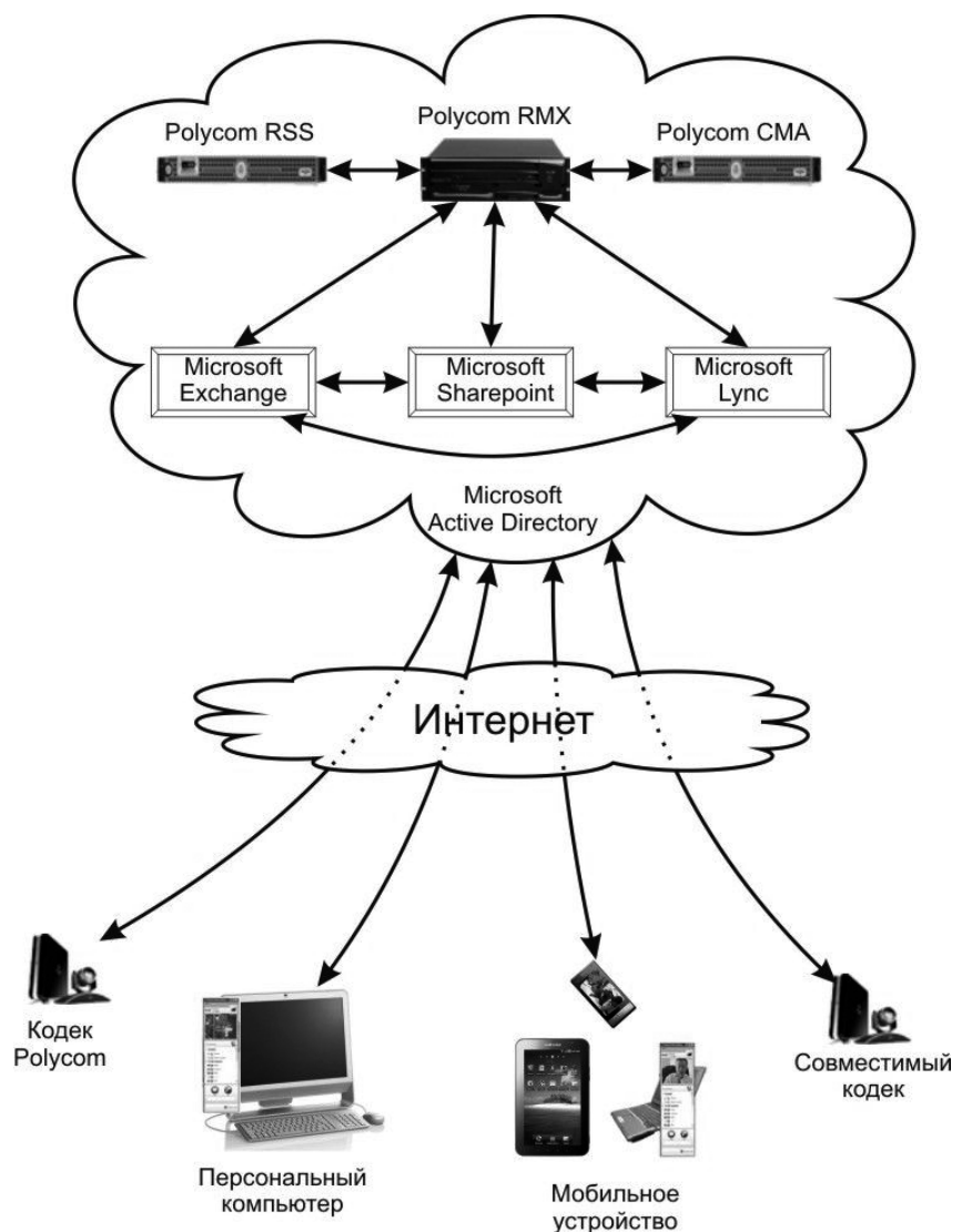
Рис. 5. Общая технологическая схема виртуальной научно-образовательной среды
