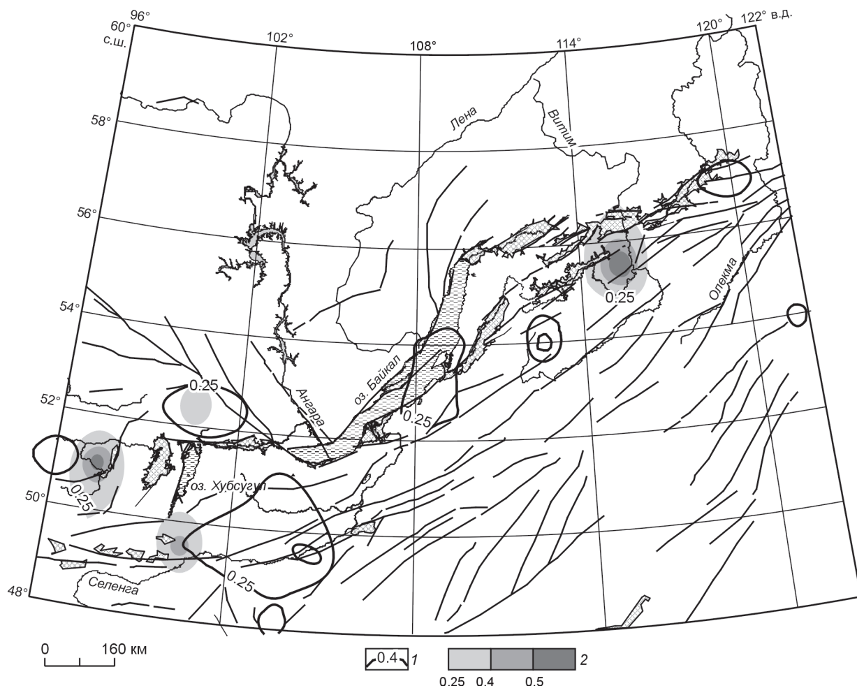
Рис. 5. Карты изолиний частоты реализации толчков-взбросов P_R , полученные по данным о фокальных механизмах и сейсмических моментах толчков.
