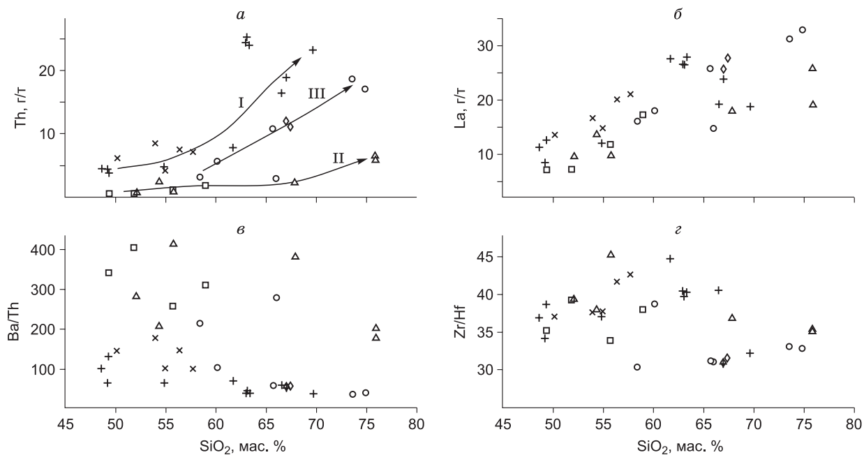
Рис. 11. Диаграммы зависимости содержаний Th ( a ), La ( б ), отношений Ba/Th ( в ) и Zr/Hf ( г ) от кремнекислотности для вулканитов УМВП и ОЧВП.
