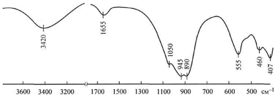
Рис. 2. ИК-спектр быковаита.
