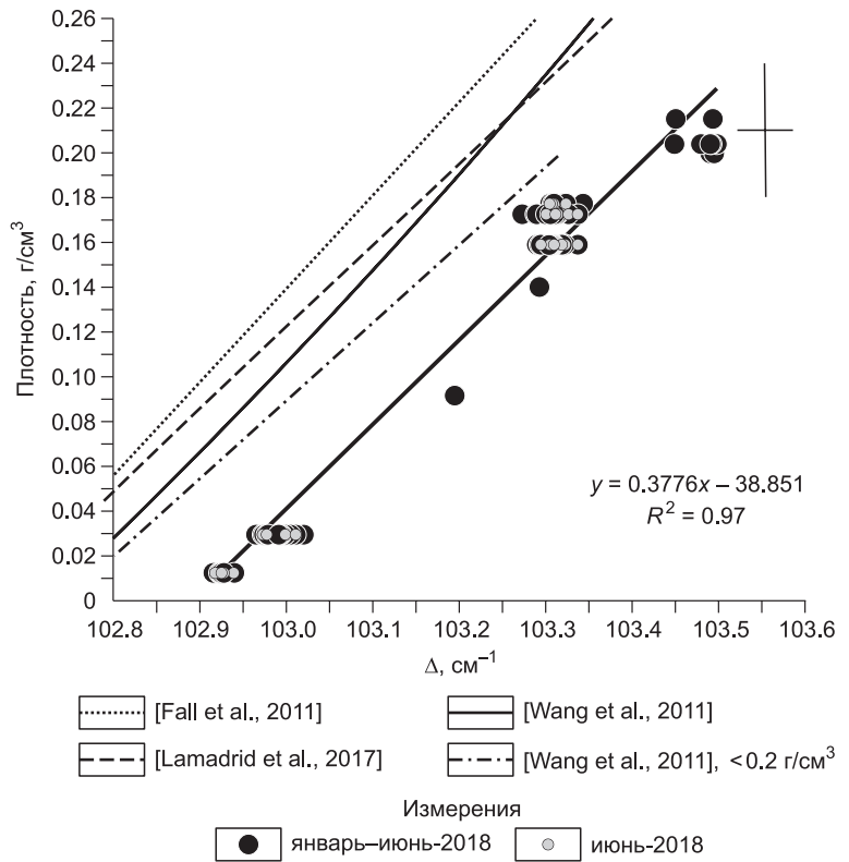
Рис. 3. Калибровочная линия для оценки плотности \text{CO}_2 в газовых пузырьках расплавных включений в зависимости от расстояния между характеристическими пиками \text{CO}_2 (диадами Ферми).
