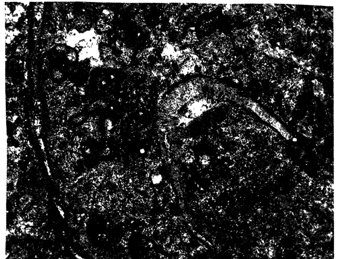
Рис. 6. Известняк детритовый
