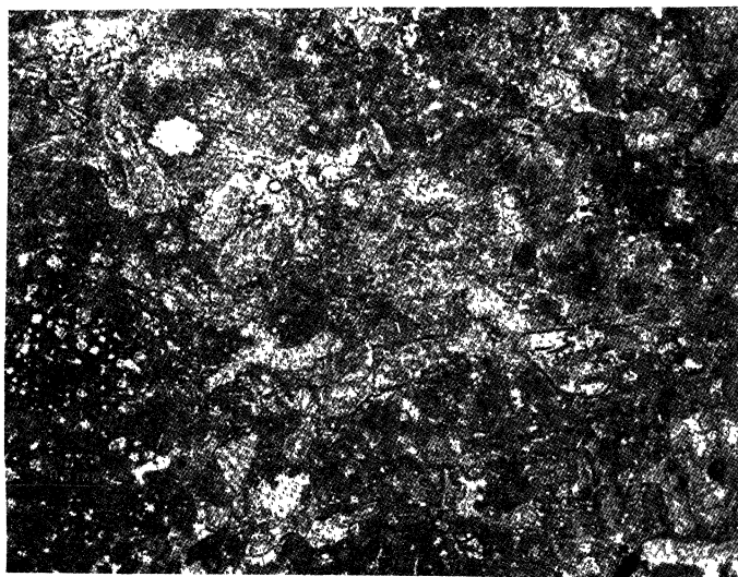
Рис. 1. Известняк водорослевый
