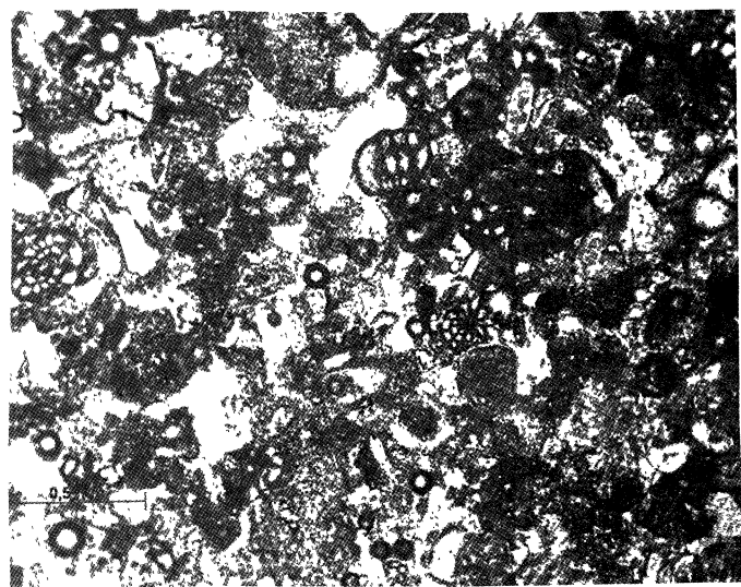
Рис. 3. Известняк водорослево-фораминиферовый
