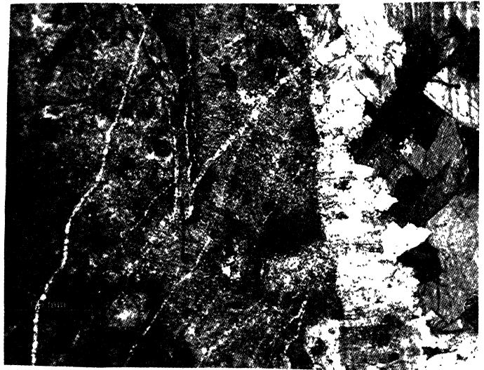
Рис. 5. Известняк водорослево-фораминиферовый (система трещин)
