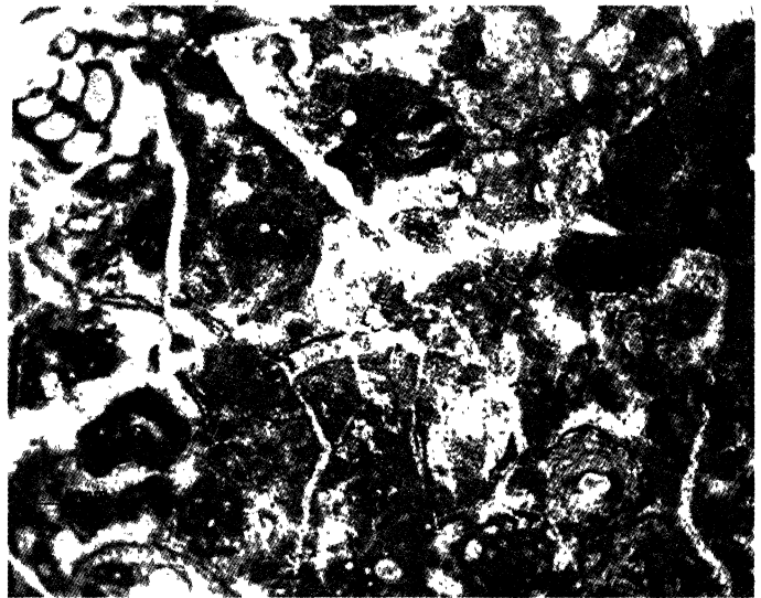
Рис. 4. Известняк водорослево-фораминиферовый
