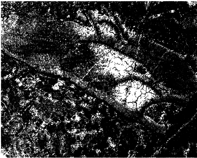
Рис. 7. Известняк микрозернистый
