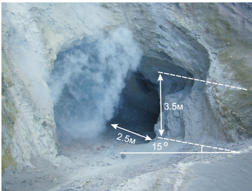
Рис. 10. Эруптивное жерло в Активной воронке Северного кратера. Фото Л.В. Котенко.
