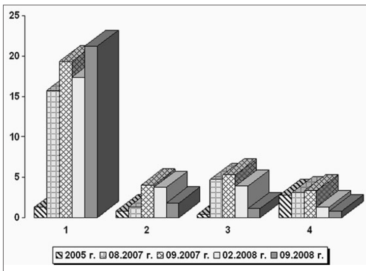
Рис. 4. Гистограмма изменения прогностических отношений газовых компонентов в 2005-2008 гг. (фумарольное поле Июльское): 1 – S/Cl, 2 – H 2 S/SO 2 , 3 – H 2 O/CO 2 × 10 -2 , 4 – S/C.
