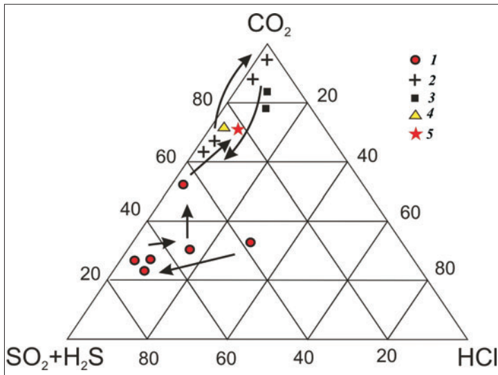
Рис. 3. Диаграмма химического состава фумарольных газов вулкана Эбеко в апреле 2009 г.: 1 – поле Июльское, 2 – Северо-Восточное, 3 – Юго-Восточное, 4 – Активная воронка, 5 – эруптивные (Меняйлов и др., 1992) и поле Июльское в апреле 2009 г. Стрелками обозначено изменение состава газов во времени.
