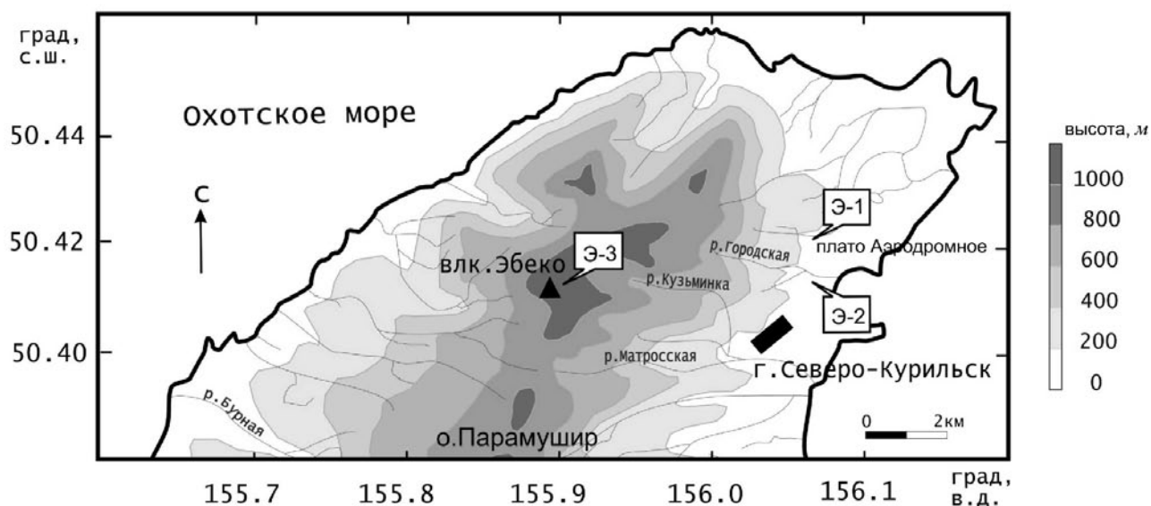
Рис. 1. Схема расположения вулкана Эбеко и точек отбора проб пепла (Э-1, Э-2, Э-3) извержения 2009 г.
