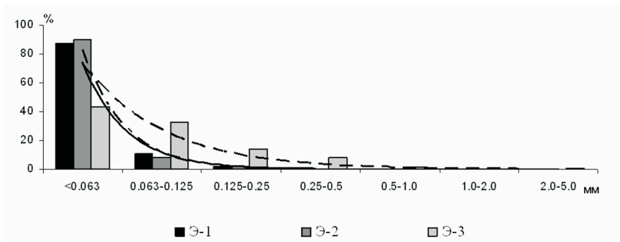
Рис. 12. Гистограмма распределения тефры извержения 2009 г. по фракциям.
