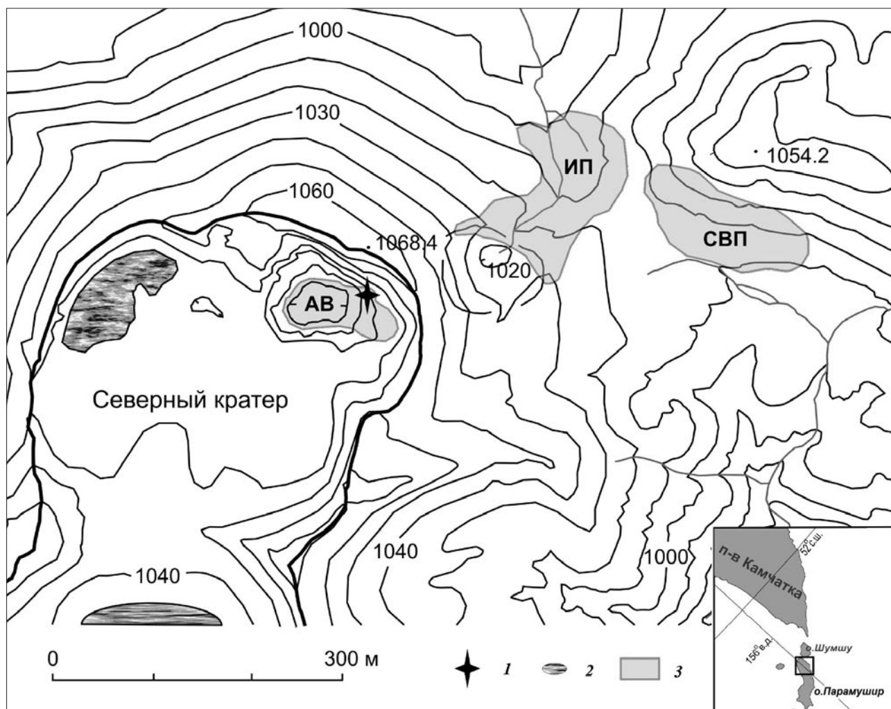
Рис. 2. Северный кратер вулкана Эбеко с прилегающим районом (по В.Н. Двигало (1989) с дополнениями авторов): АВ – Активная воронка, ИП – фумарольное поле Июльское, СВП – Северо-Восточное фумарольное поле, 1 – эруптивное жерло, 2 – кратерные озера, 3 – площади термальных полей.
