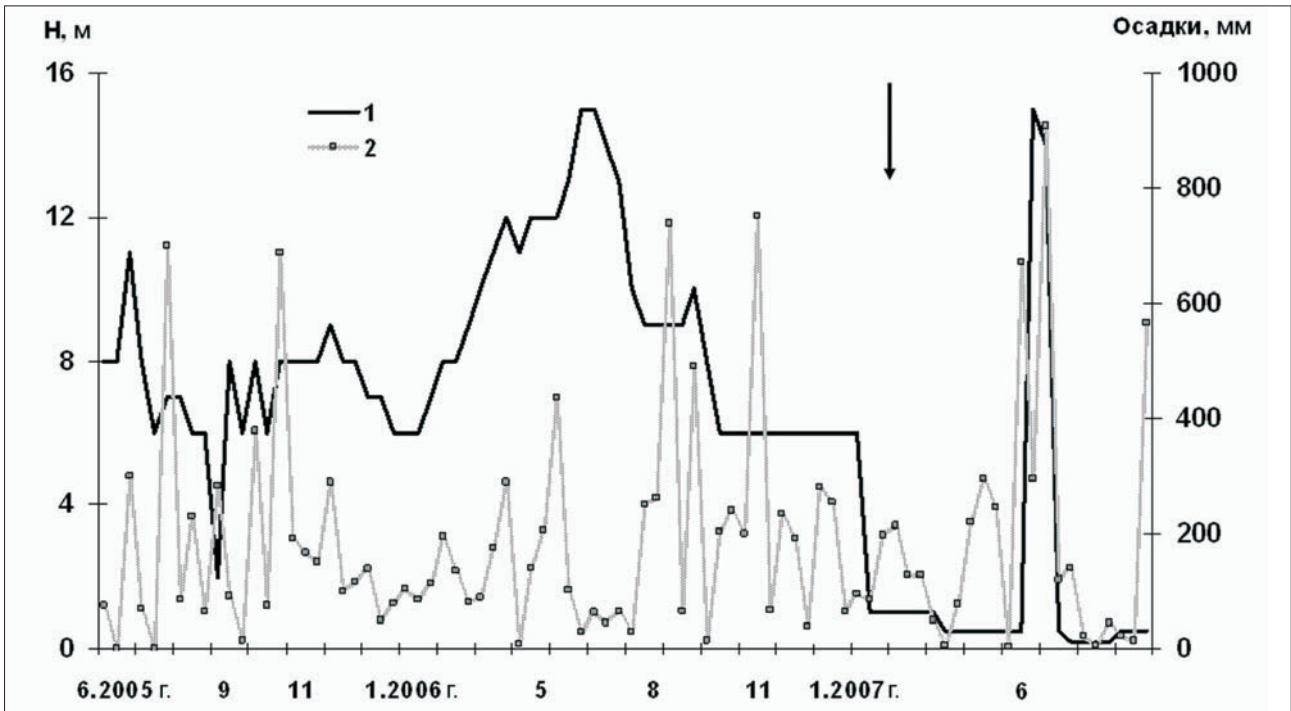
Рис. 6. График изменения глубины озера (1) в Активной воронке и декадных сумм осадков на уровне кратера (2). Стрелкой обозначен взрыв 16.02.2007 г.
