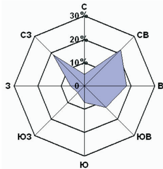
Рис. 11. Ориентация пепловых шлейфов за весь период извержения вулкана (повторяемость в % от общего числа случаев).
