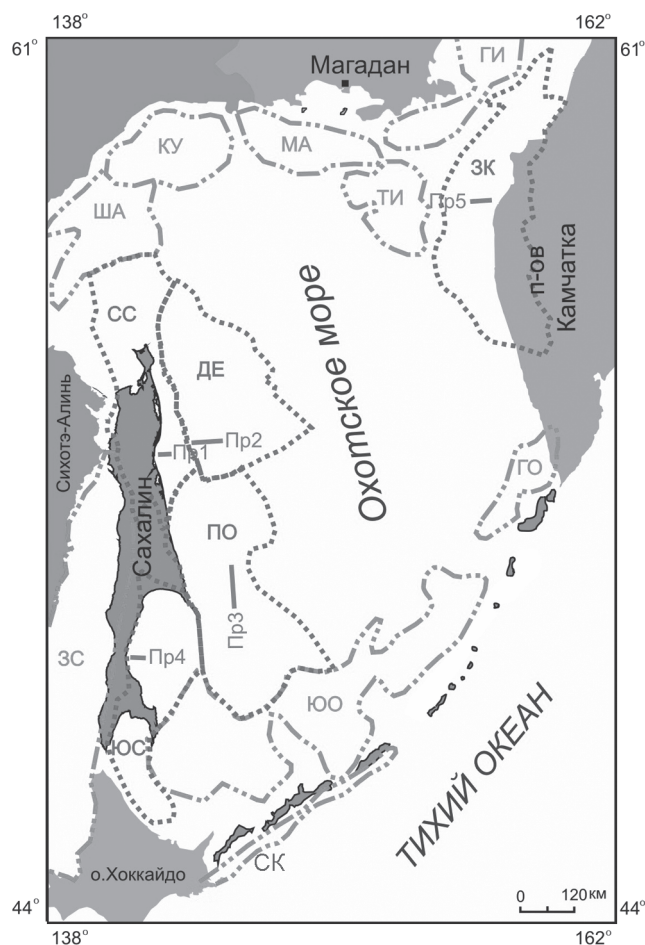
Рис. 2. Обзорная схема и кайнозойские осадочные бассейны Охотоморского региона.
