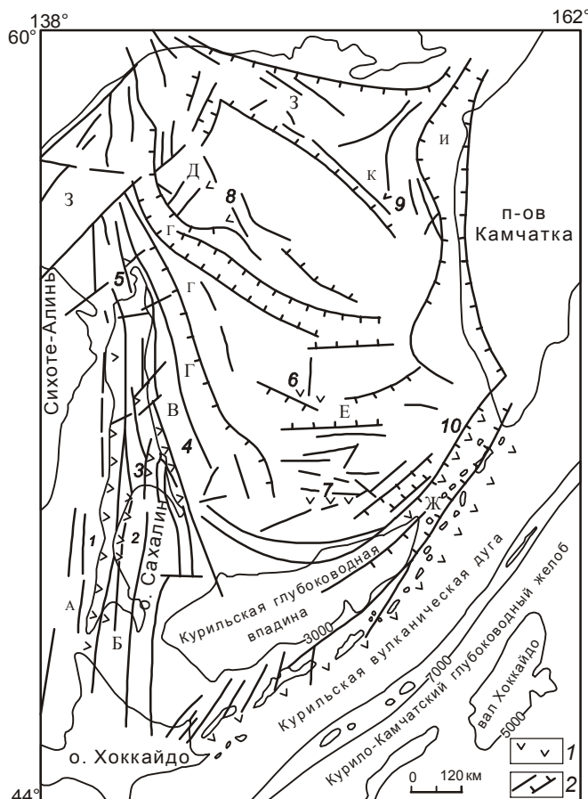
Рис. 1. Тектоническая схема Охотоморского сектора кайнозойской активной окраины Пацифика [9].
