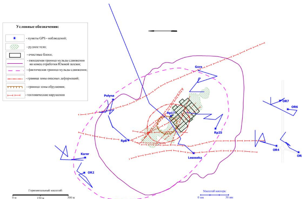
Рис. 3 – Векторы горизонтальных сдвижений реперов геодинамического полигона
