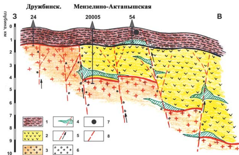
Рис. 1. Схема миграции подвижных веществ юго-западной бортовой части Камско-Бельского авлакогена. 1 – фанерозой; 2 – верхний протерозой; 3 – кристаллический фундамент; 4 – интрузивные тела основного состава; 5 – возможное направление миграции; 6 – предполагаемые проницаемые зоны; 7 – нефтенасыщение; 8 – разломы.
