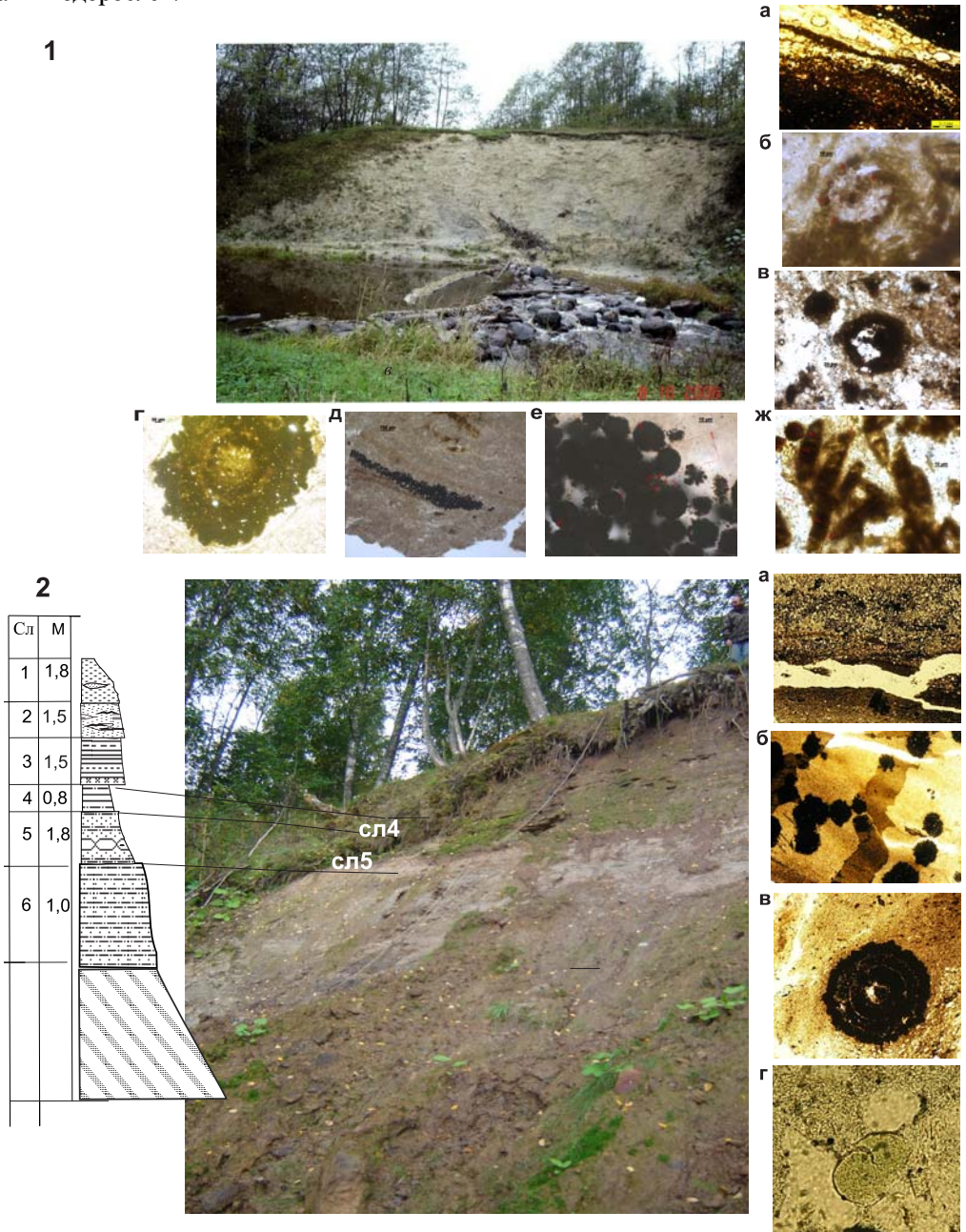
Рис. 2. Разрезы отложений котлинского горизонта: 1 – василеостровской свиты на р. Черная (II). а – цианобактериальные маты; б – Siphonophycus Kestron Schopf, 1968; в – Paleo Palaeolynghya cf. P. Basghoortiana , г, д, е – пирит по колониям цианобактерий, ж – Oscillatoria aff. O. meding . 2 – воронковская свита на р. Воронка (B-1): а – слои алевролита сменяются слоями алевритистой глины; б – глина алевролитистая с ходами илеодов и железистыми включениями; в – железистые включения; г – глобулы глауконита в песчанике.
