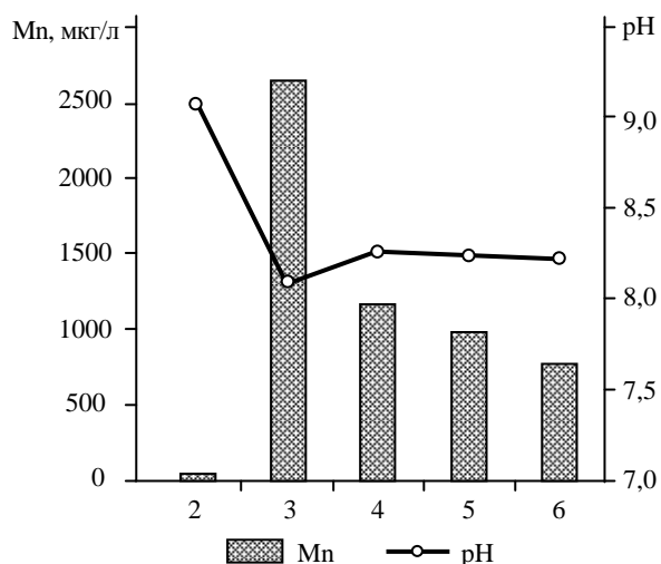
Содержание марганца и изменение pH в исследуемых водных объектах по мере удаления от источника 2-6 – номера проб
