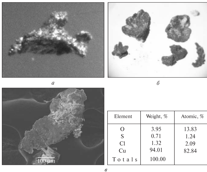
Рис. 5. Изогнутые, пластинчатые зерна серебра ( a ) и меди ( б, в ) из аллювиальных отложений Днепра: a, б — карьер на первой надпойменной террасе южнее острова Вербки. Бинокляр, ув.: a — 180 X ; б — 50 X ; в — пластинчатое выделение самородной меди с выцветами вторичных карбонатов меди; п. Каланчак, поисковая скв. гл. 11 м. РЭМ, МЗА
