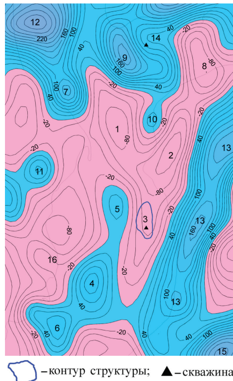
Рис. 2. Карта аномалий магнитного поля \Delta T : цифрами обозначены минимумы и максимумы \Delta T_{ср}
