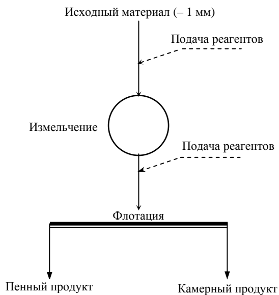
Технологическая схема проведения опытов
