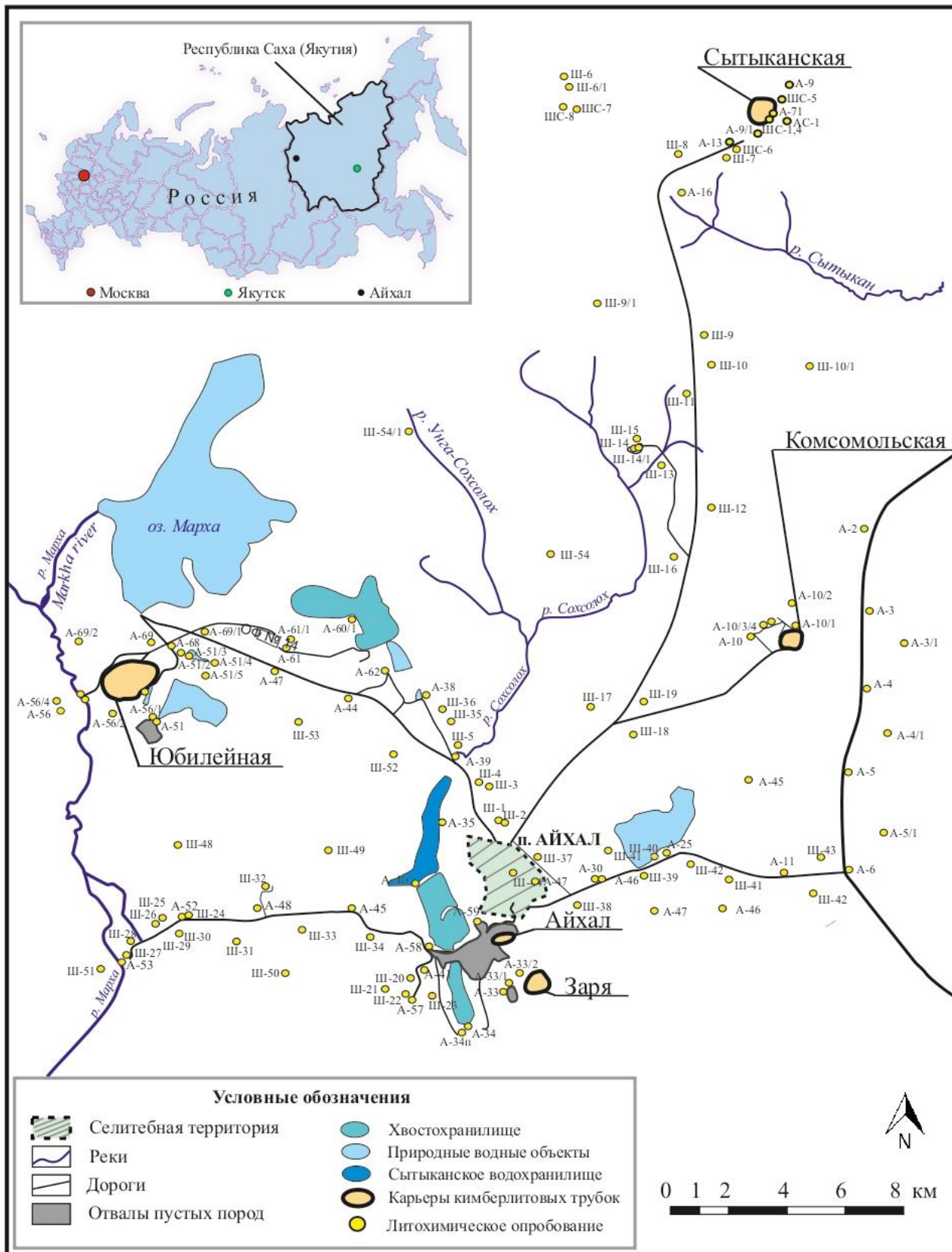
Рис. 1. Схема опробования территории исследования
