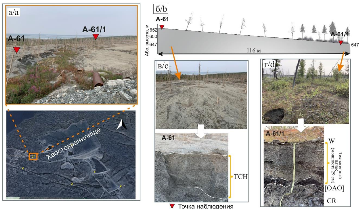
Рис. 2. Почвенный покров в зоне воздействия хвостохранилищ АГОК: (а) космоснимок с общим видом хвостохранилища ОФ № 14 и выделенным участком опробования по линии А-61–А61/1; (б) геоморфологический профиль участка по линии А-61–А61/1; (в) фото участка опробования т.н. А-61 – «свежий» нанос кимберлитового песка в результате аварийного разрыва пульповода и вертикальный профиль разреза; (г) участок опробования в т.н. А61/1 – «старый» нанос с признаками начальной стадии восстановления напочвенного покрова и вертикальный профиль разреза
