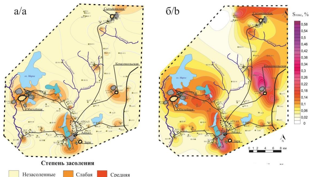
Рис. 8. Схема пространственного распространения засоления (а) и суммы токсичных солей (б) в почвах промышленной площадки АГОК
