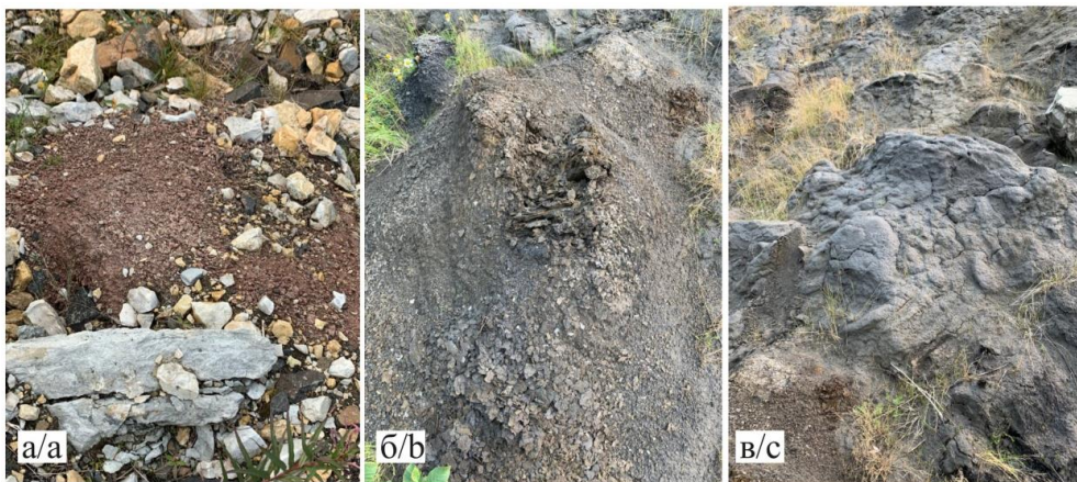
Рис. 5. Дезинтегрированные породы отвалов трубки «Юбилейная»: а) образец 922; б) образец 923; в) образец 924 Fig. 5. Disintegrated rocks from the «Yubileinaya» pipe dumps: а) sample 922; б) sample 923; в) sample 924
