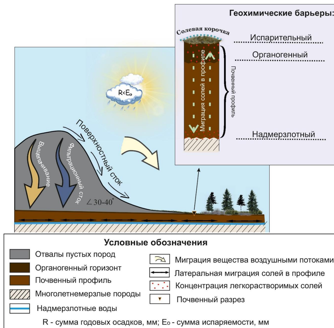
Рис. 6. Схема миграции солей в зоне воздействия отвалов пустых пород
