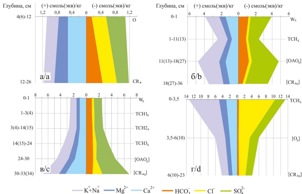
Рис. 3. Солевые профили почв промышленной площадки АГОК (а – фоновая почва; б–г – антропогенно-преобразованные почвы): а) не засоленный; б) сульфатный тип средней степени засоления; в) хлоридно-сульфатный тип средней степени засоления; г) хлоридный тип засоления с вариациями от очень сильной степени с поверхности до средней и слабой – в нижних горизонтах
