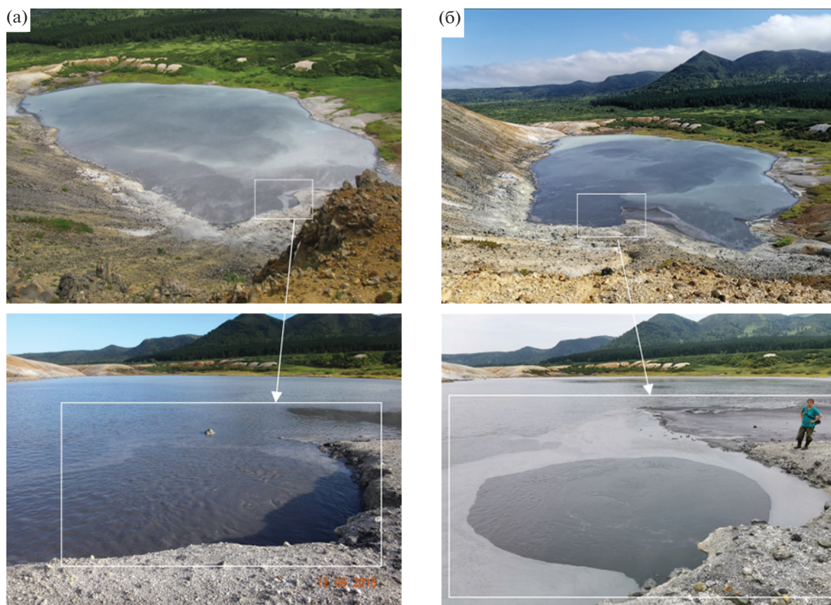
Рис. 3. Воронка с термальным потоком в северо-западной части оз. Кипящее по состоянию на сентябрь 2015 г. (а) и сентябрь 2020 г. (б).
