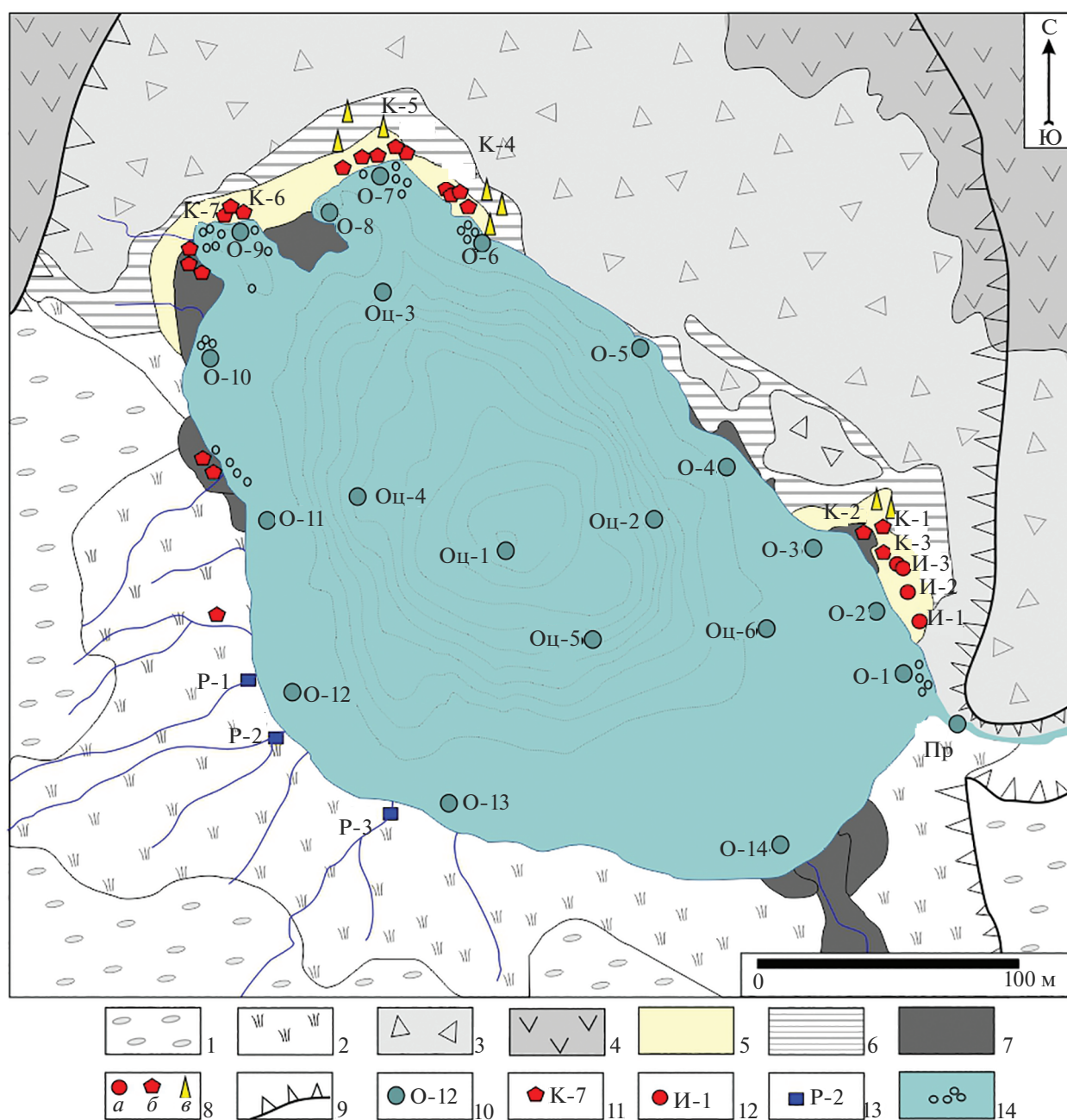
Рис. 2. Схема оз. Кипящее с точками гидрохимического опробования 2020–2021 гг. (геологическая основа – из работы [Власов, 1971]).
