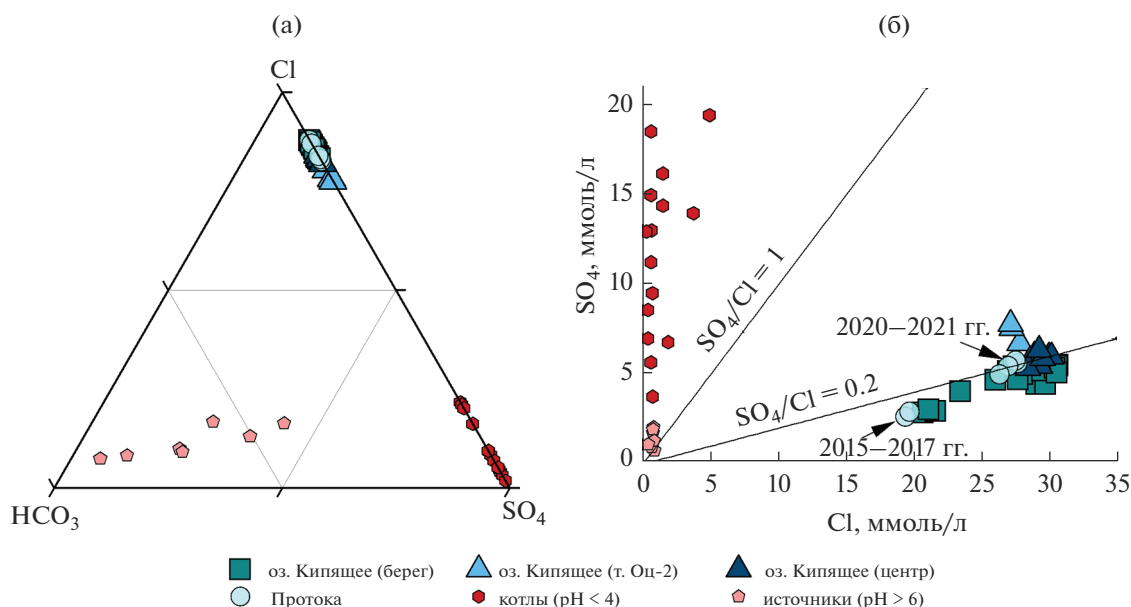
Рис. 5. Анионный состав вод оз. Кипящее и береговых термопроявлений.
