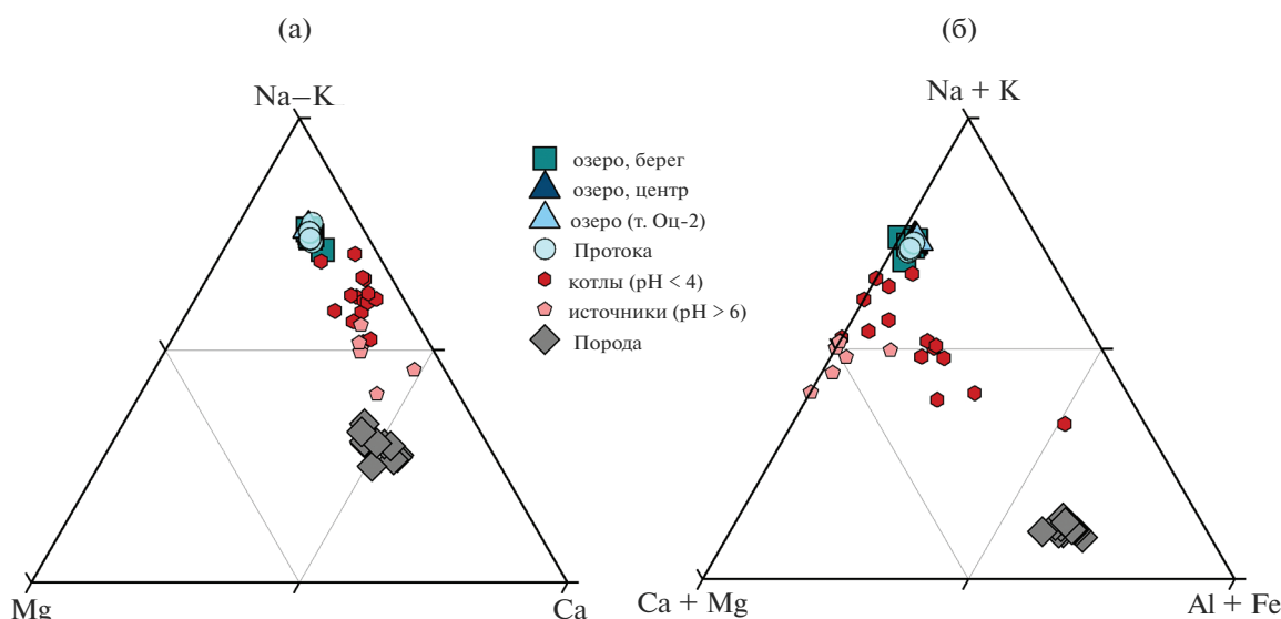
Рис. 6. Относительные концентрации катионов в воде оз. Кипящее и береговых термопроявлений. а – соотношение \text{Ca/Mg/Na + K} ; б – соотношение \text{Ca + Mg/Al + Fe/Na + K} .
