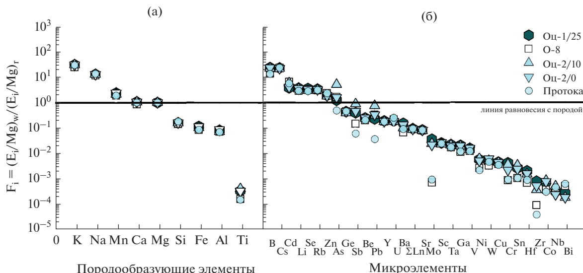
Рис. 7. Коэффициенты обогащения элементов между вмещающей породой и раствором для породообразующих (а) и редких (б) элементов оз. Кипящее.
