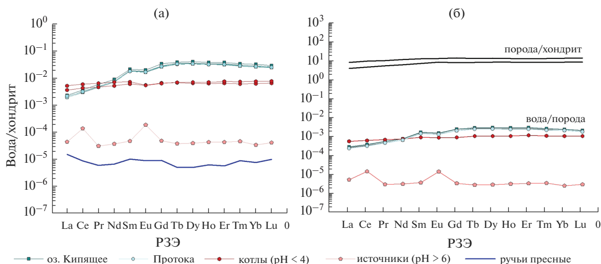
Рис. 8. Нормированные профили РЗЭ в разных типах вод в районе оз. Кипящее по отношению к хондриту, по [McDonough, Sun, 1995] (а) и вмещающим породам, по [Мартынов и др., 2010] (б).
