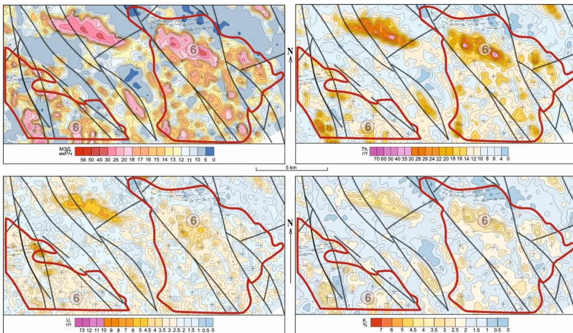
Рис. 7. Радиогеохимические поля Чиримбинского массива Fig. 7. Radiogeochemical fields of the Chirimbinsky massif
