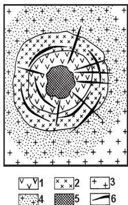
Рис. 25. Общая схема строения карбонатитового месторождения: 1 – щелочные породы; 2 – ультраосновные породы; 3 – гнейсы; 4 – фениты; 5 – шток карбонатитов; 6 – жилы карбонатитов. (Кузнецов, Ситдикова, метод. пособие, 2008).
