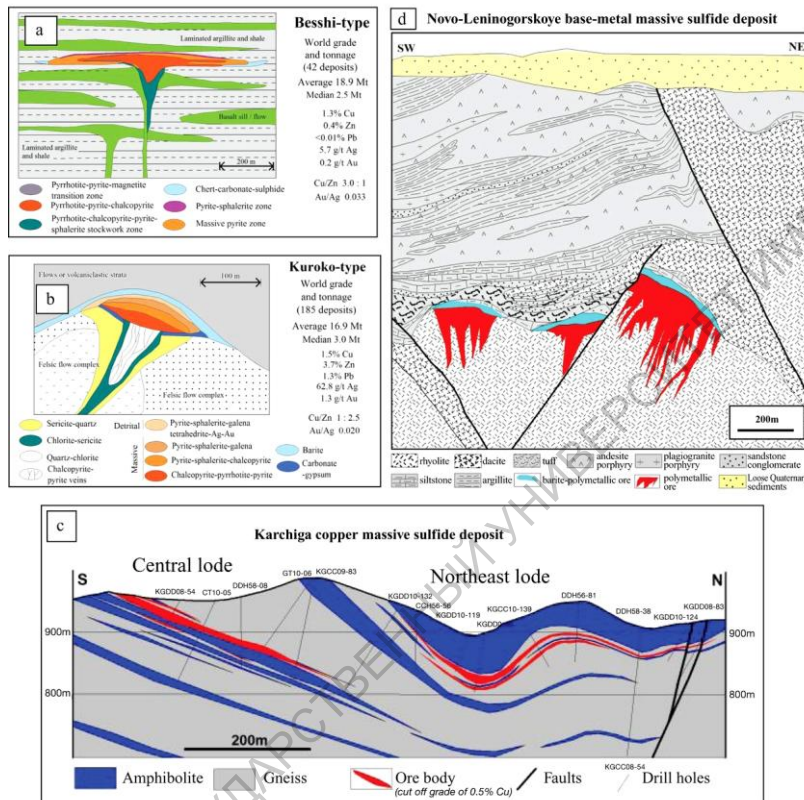
Рис. 59. Сравнение структур медноколчеданного месторождения Карчига, Юго-Зап.Алтай (с) и колчеданно-полиметаллического месторождения Ново-Лениногорское, Рудный Алтай (d), как представителей типов Бесши и Куроко (a,b). По Лобанову К.В., 2012.
