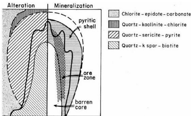
Рис. 65 (Fig. 1.3 на рис.64). Типичная зональность околорудных пород и рудной залежи медно-порфирового месторождения ( http://pacmag.com.au/faqs.11.html )
