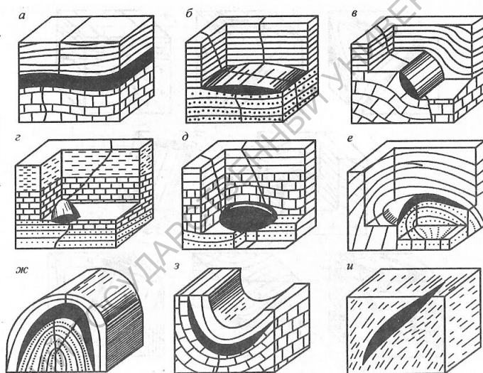
Рис. 10. Согласные рудные тела. По А.В.Королеву, П.А.Шехтману (Милютин А.Г., 2008). а - рудный пласт; б - рудная залежь; в - рудная лента; г - брусковидное тело; д - рудное гнездо; е - куполовидная залежь; ж - седловидная залежь; з - желобовидная залежь; и - флексурная залежь (линза).
