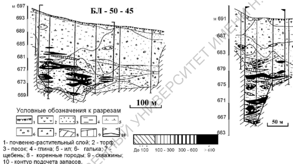
ПЛАН РОССЫПИ С ИЗОСОДЕРЖАНИЯМИ ЗОЛОТА СХЕМА ИЗУЧЕННОСТИ (по материалам Н.Б. Трубникова, 1980)
