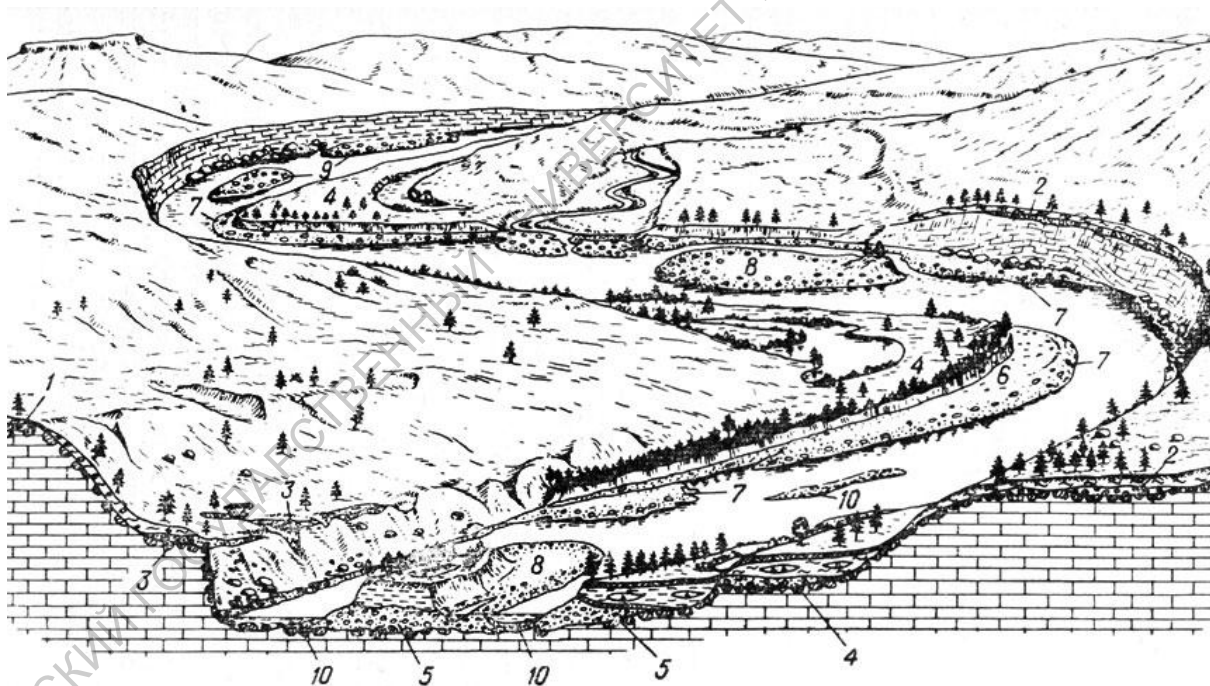
Рис. 78. Схема расположения россыпей различных типов в долине реки (по А. П. Бобричеву и др.). Террасовые россыпи: 1 - террасы 5, 2 - террасы 4, 3 - террасы 3, 4 - террасы 2, 5 - террасы 1. Долинные россыпи: 6 - пойменные, 7 - береговых отмелей, бечевников, 8 - шлейфовые размываемых террасовых останцов, 9 - косовые, 10 - собственно русловые.
