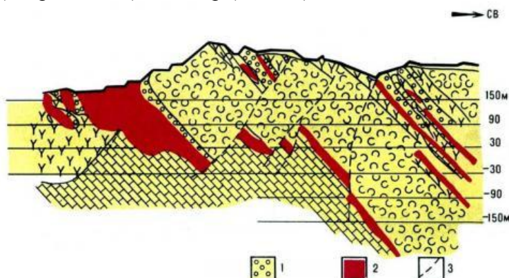
Рис. 34. Схематизированная модель строения Соколовско-Сарбайских скарновых месторождений. Кустанайская обл., Казахстан. 1 - скарны; 2 - магнетитовые руды; 3 - сбросы.
