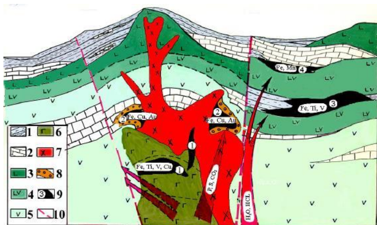
Рис. 32. Идеализированная схема размещения скарновых магнетитовых месторождений в вулcano-плутонической структуре. 1 – терригенно-карбонатные отложения; 2 – известняки; 3-5 – породы вулканической серии: 3 – эффузивы и их туфы, преимущественно базальтового состава, 4 – то же андезито-базальтового состава, 5 – то же андезитового состава; 6-7 – интрузивный комплекс, комагматичный вулканитам: 6 – габбро, габбро-диориты, 7 – диориты, кварцсодержащие диориты, диорит-порфиры; 8 – пироксен-гранатовые скарны; 9 – магнетитовые месторождения и их подтипы (цифры в кружочках): 1 – магнетитовые позднемагматические, 2 – собственно скарновые, 3 – скаполитовые, 4 – гидросиликатные; 10 – разрывные нарушения ( http://www.uran.ru/structure/institutions/igg/Publications/Prokin/stat41.htm )
