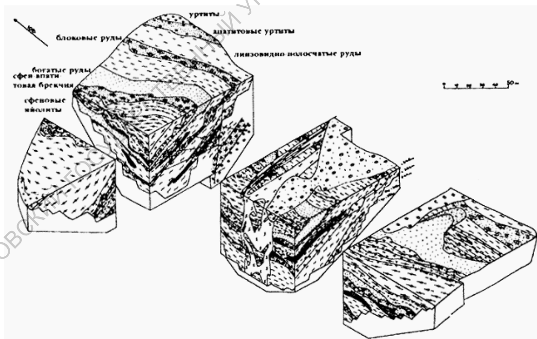
Рис. 22. Геологическое строение Кукивумчоррского апатитового месторождения (по С.В.Синогейкину). http://geo.web.ru/db/msg.html?mid=1171483&uri=img2.htm
