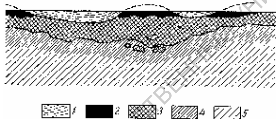
Рис. 73. Типовой разрез площадной коры выветривания по серпентинитам. 1 -наносы; 2 - охры и бурые железняки латеритного горизонта (кобальтоносные); 3 - нонтрониты (никеленосные монтмориллониты) нонтронитового горизонта; 4 - нонтронитизированные серпентиниты, переходящие книзу в магнетитоносные и опализованные серпентиниты; 5 - неизмененные серпентиниты.
