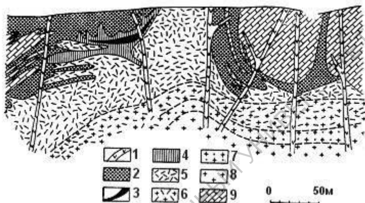
Рис. 39. Схематический поперечный геологический разрез грейзенового месторождения в известняках у контакта с гранитом. (по И. Говорову). 1 - порфириитоиды; 2 - слюдисто-флюоритовые грейзены; 3 - диаспор-топаз-флюоритовые грейзены; 4 - топаз-флюоритовые грейзены; 5 - кварц-топазовые грейзены; 6 - сильно грейзенизированные граниты; 7 - умеренно грейзенизированные граниты; 8 - слабо грейзенизированные граниты; 9 - известняки.
