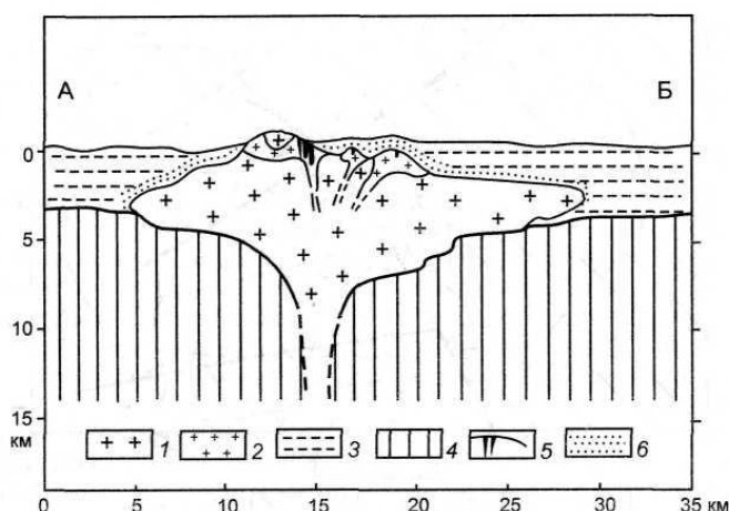
Рис. 38. Схематический продольный геологический разрез Акчатауского гранитного плутона. 1 - крупнозернистые граниты I фазы; 2 - средне- и мелкозернистые граниты фаз II и III; 3 - терригенные и вулканогенные вмещающие породы; 4 - кристаллические породы докембрийского фундамента; 5 - рудные тела; 6 - контактовые роговики.
