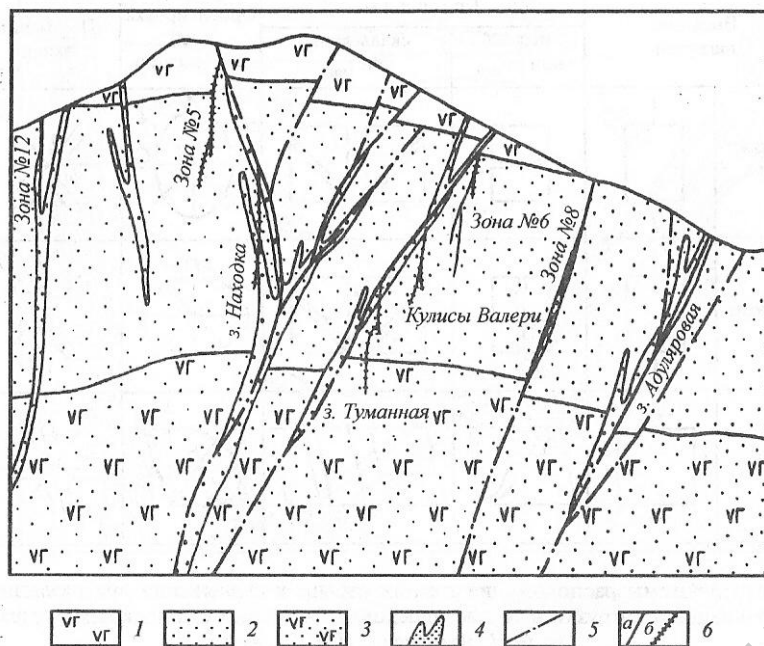
Рис. 8. Разломы и рудоносные зоны Агинского золоторудного месторождения. Камчатка. По Б.В.Гузману (Милютин А.Г., 2008). 1 - андезито-базальты; 2 - туфы и туфобрекчии; 3 - туфы андезито-базальтов; 4 - дайки; 5 - сбросо-сдвиги; 6 - рудоносные жилы (а) и зоны прожилков (б).
