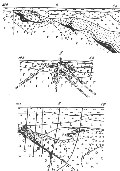
Рис. 52. Геологические разрезы вулканической постройки Юбилейного месторождения. Рудные залежи локализованы в зоне контакта базальтовых (внизу) и риолитовых толщ контрастной формации Ирендыкской палеодуги (ю.Урал). 1 - риолиты (а) и рио-дациты (б); 2 - дациты (а) и андезито-дациты (б); 3 - магматические брекчии: автомагматические (а) и эксплозивные (б); 4 - границы экструзивных тел (а) и их внутренних зон (б); 5 - четвертичные рыхлые отложения.
