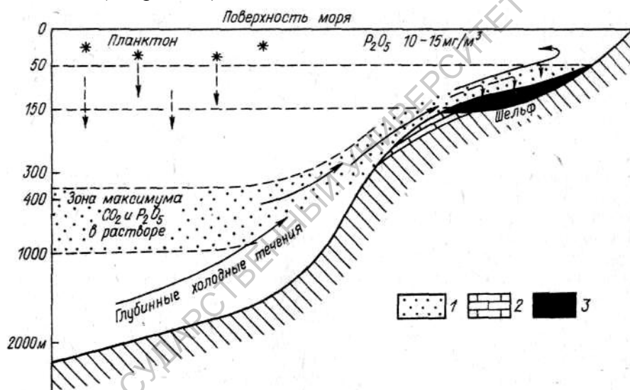
Рис. 85. Схема фосфоритообразования в зоне шельфа по хемогенной модели А. В. Казакова. / — морские воды, обогащенные \text{CO}_2 и \text{P}_2\text{O}_5 ; 2 — осадки глинисто-известковой фации; 3 — осадки фосфоритной фации.
