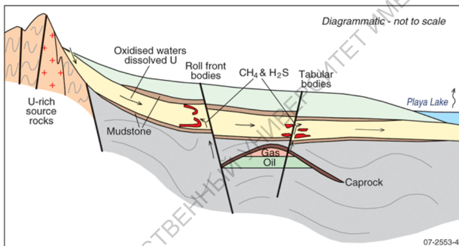
Рис. 91. Схематический разрез, объясняющий формирование инфильтрационных и эксфильтрационных месторождений. ( http://www.stockhouse.com/bullboards ).
