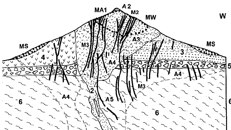
Рис. 40. Оловянно-серебряное месторождение Потоси, Боливия (По Силлитое и др., 1998 и Бартос, 2000). Условные обозначения: MA1 - привершинный "козырек" кавернозного остаточного микрокварцита; MW - обогащенная серебром зона окисления; M2 - Рой жил и прожилков Ag-Sn минерализации в измененном порфире; M3 - положение зоны высоко продвинутой зоны трещин с прожилками Ag, Sn, Pb, Sb, As, расширяющихся на верхнем уровне и окруженных вкрапленностью касситерита; A: Зоны минеральных изменений: A1 - кремнезем опализации; A2 - джаспероиды; A3 - зона аргиллизации; A4 - серицит-пиритовая зона; A5 - кварц-турмалиновая зона; 2. Купол дацитовых порфиров, переходящих в брекчии; 3 - туфы, 4 - вулканогенно-обломочные породы; 5. Эксплозивные брекчии; 6. Филлиты; MS - каменистые осыпи с обломочным касситеритом.
