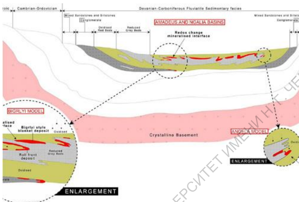
Рис. 90. Модели формирования урановых месторождений в артезианских бассейнах (Sectional Model of Ngalia and Amadeus Basin uranium mineralisation models).
