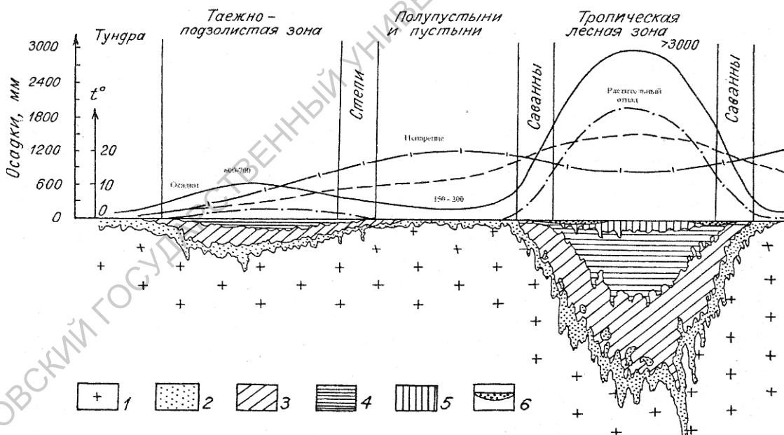
Рис. 75. Зависимость глубины и степени выветривания горных пород от суммы ежегодных осадков и среднегодовой температуры в различных ландшафтно-климатических зонах (по Н.М.Страхову). 1 - неизменные породы; 2 - зона дресвы, химически мало измененной; 3 - гидрослюдисто-каолинитовая (монтмориллонитовая) зона; 4 - каолинитовая (монтмориллонитовая) зона; 5 - зона охр и гиббсита - латеритный горизонт; 6 - латеритный "панцырь" (плита бурых железняков).
