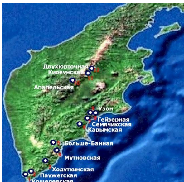
Рис. 67. Геотермальные и гидротермальные системы Камчатки (по Сугробову В.М., 1995).
