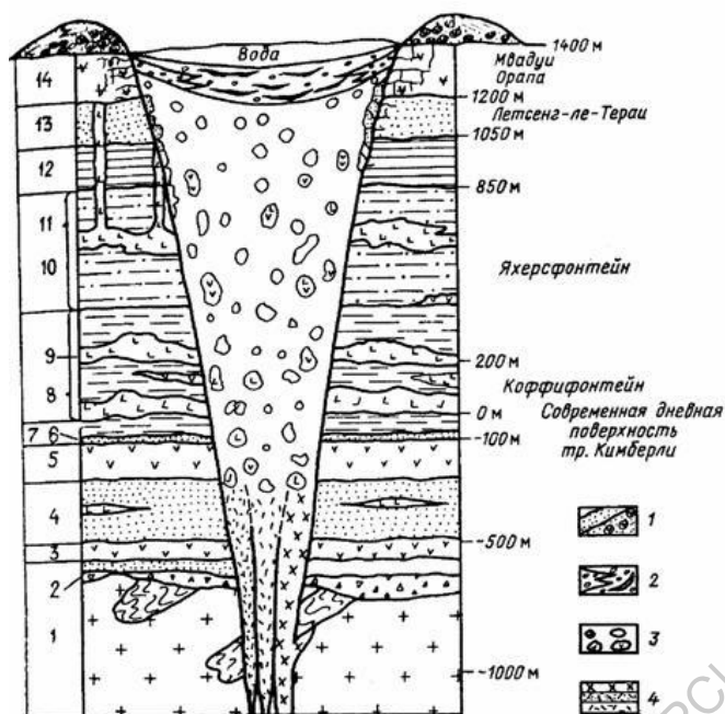
Рис. 20. Модель кимберлитовой трубки (по Дж. Хоторну): 1 - выброшенный туфовый материал; 2 - разнозернистые осадки кратерного озера; 3 - агломератовый туф; 4 - разновидности интрузивных брекчий; 1 - первичная система (древние гранитогнейсы и сланцы); 2-5-система Вентерсдорп: 2-конгломераты р. Вааль, 3 - кварцевые порфиры, 4 - кварциты, 5 - андезитовые лавы; 6-14-система Карру: 6 - сланцы и тиллиты Двайка, 7, 9, 10 - долериты Карру, 1 - сланцы Эка, 11-свита Босфорт, 12 - красные слои, 13 - пещерный песчаник, 14 - лавы Стормберг ( http://niigiger.narod.ru/predl.html )
