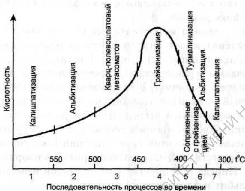
Рис. 36. Схема эволюции кислотности и температуры послемагматических растворов
