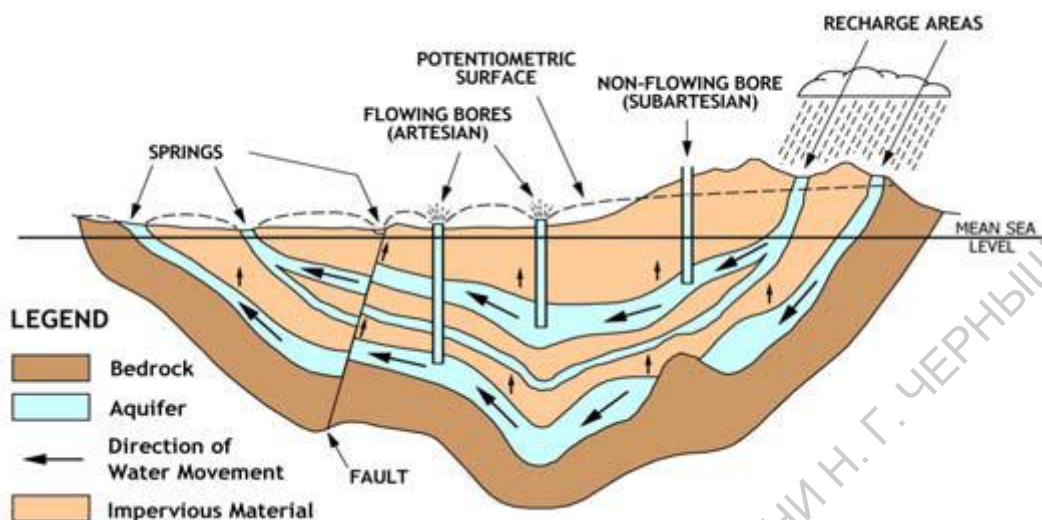
Рис. 86. Упрощённое строение Великого артезианского бассейна, Австралия http://www.derm.qld.gov.au/factsheets/pdf/water/w68.pdf
