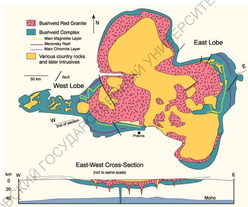
Рис. 18. Комплекс Бушвельд
