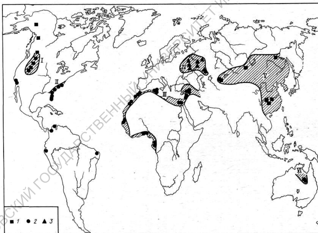
Рис. 84. Фосфоритоносные провинции мира. Месторождения фосфоритов: 1 — микрозернистых, 2 — зернистых, 3 — желваковых. Провинции: I — Скалистых гор, II — Восточно-Американской береговой равнины, III — Аравийско-Африканская, IV — Русской платформы, V — Азиатская, VI — Австралийская.
