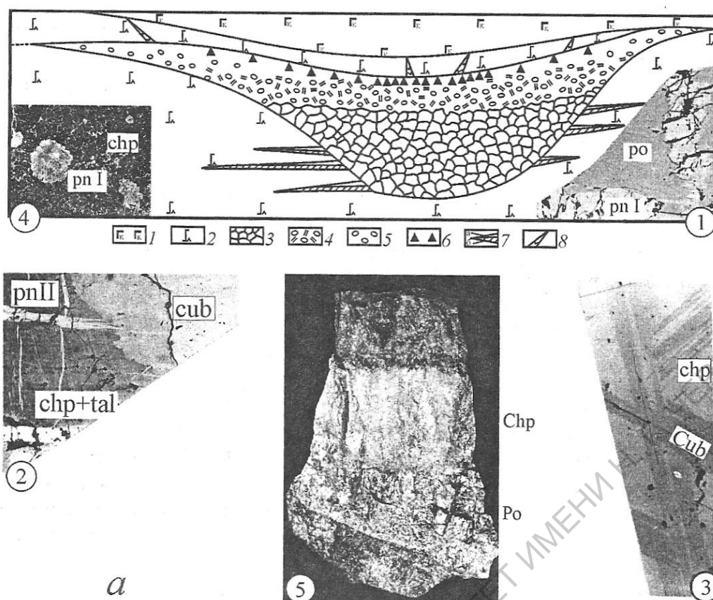
Рис. 17. Схематизированный разрез рудной залежи и типы руд месторождения Норильск I (по А.П.Лихачеву, 2006). 1 - контактовый габбро-долерит интрузии Норильск I; 2 - базальтовый порфирит; 3 - пирротин-пентландитовая ассоциация; 4 - пентландит-кубанит-халькопирит-талнахитовая ассоциация; 5 - пентландит-халькопиритовая ассоциация; 6 - магнетитовая минерализация; 7 - сульфидные ответвления от пирротиновой зоны, дифференцированные на существенно халькопиритовую (а) и существенно пирротиновую (б) части (см. вставку 5); 8 - ответвления пироксен-полевошпатового состава (в кровле залежи). Цифры в кружках: вставка 1 - пентландит-пирротиновая ассоциация, \times 45 ; вставка 2 - пентландит-кубанит-халькопирит-талнахитовая ассоциация, \times 150 ; вставка 3 - кубанит-халькопиритовая ассоциация, \times 350 ; вставка 4 - пентландит-халькопиритовая ассоциация, уменьшено в 1,5 раза; вставка 5 - фрагмент ответвления от сульфидной залежи, дифференцированный на нижнюю пирротиновую и верхнюю халькопиритовую части, в натуральную величину.
