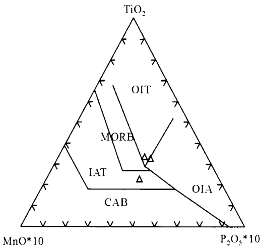
图8 塔尔浪斜长角闪岩 TiO 2 -MnO-P 2 O 5 判别图 (Pearce and Cann, 1973) (图中: CAB-大陆弧玄武岩; MORB-洋中脊玄武岩; IAT-岛弧拉斑玄武岩; OIT-洋岛拉斑玄武岩; OIA-洋岛碱性玄武岩)
