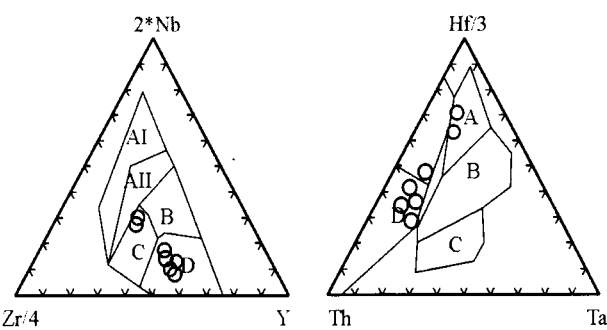
图 9 塔尔浪辉长岩 Zr-Nb-Y 判别图(Meschede, 1986)和 Hf-Th-Ta 判别图(Wood, 1980)(其中 Zr-Nb-Y 判别图中: A I 区为板内碱性玄武岩, A II 区为板内碱性玄武岩和板内拉斑玄武岩, B 区为 E 型 MORB, C 区为板内拉斑玄武岩和火山弧玄武岩, D 区为 N 型 MORB 玄武岩和火山弧玄武岩。其中 Hf-Th-Ta 判别图中, A 区为 N 型 MORB, B 区为火山弧玄武岩, C 区为板内碱性玄武岩, D 区为岛弧拉斑玄武岩( Hf/Th > 3.0 )和钙碱性玄武岩( Hf/Th < 3.0 ))
