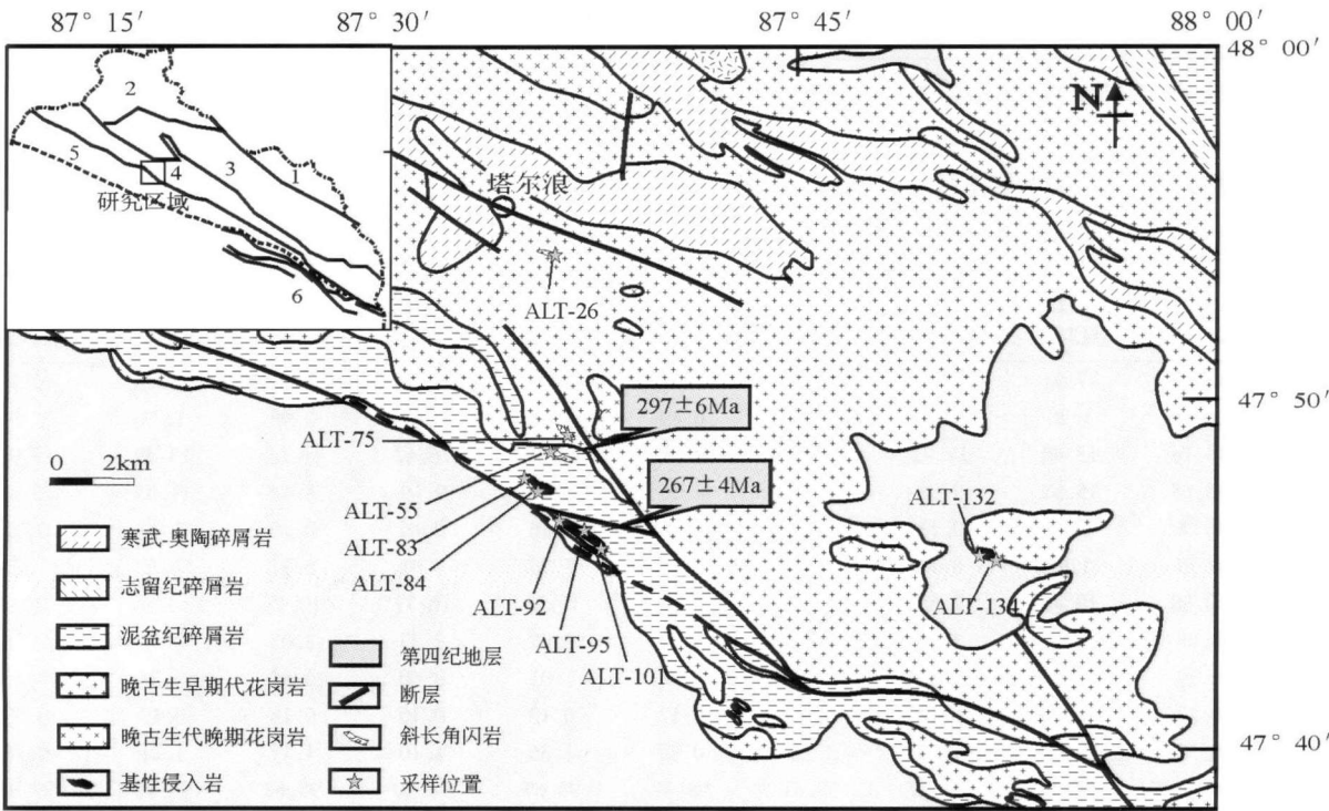
图 1 塔尔浪地区地质图 Fig. 1 Simplified geological map of Tarlang region
