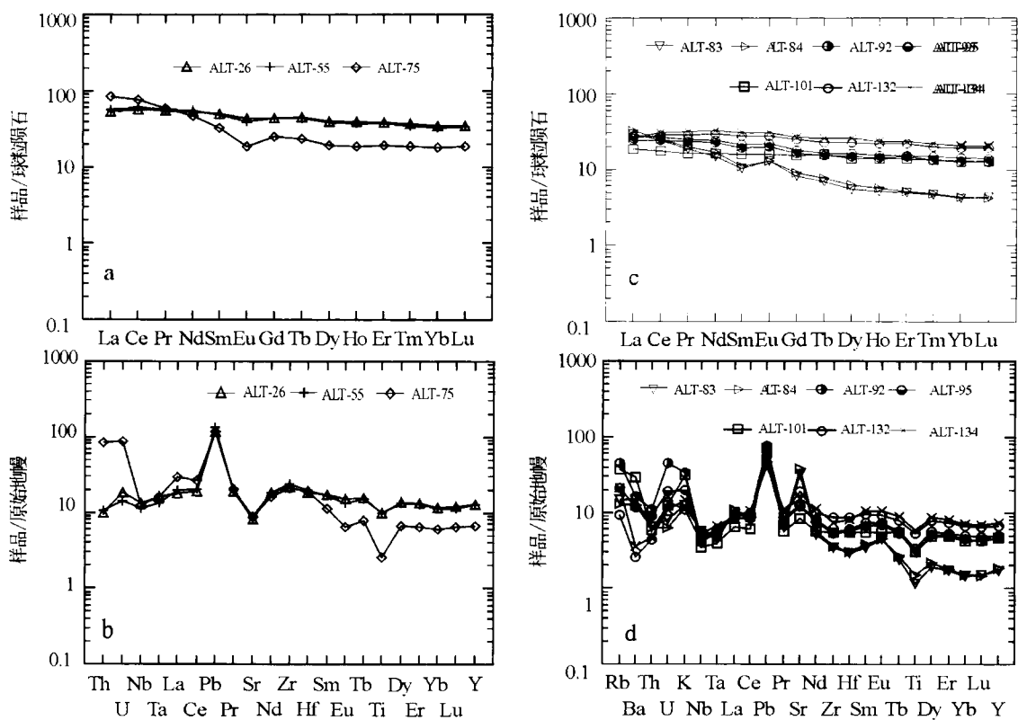
图7 球粒陨石标准化稀土元素分配图及原始地幔标准化微量元素蛛网图(球粒陨石及原始地幔标准化值引自 Sun and McDonough,1989)
