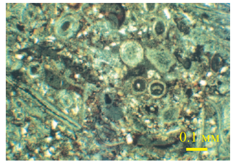
Рис. 8. Известняк органо-генно-детритовый, мианково-криноидно-брахиоподовый. Обнажение у с. Борок, казанский ярус, байтуганские слои, пачка «средне-спириферовый известняк». Концентрация свободных органических радикалов I типа = 2 \times 10^{13} spins/g.
