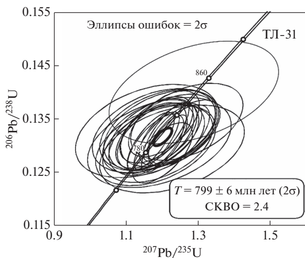
Рис. 9. Диаграмма с конкордией для цирконов из туфов (ТЛ-31).
