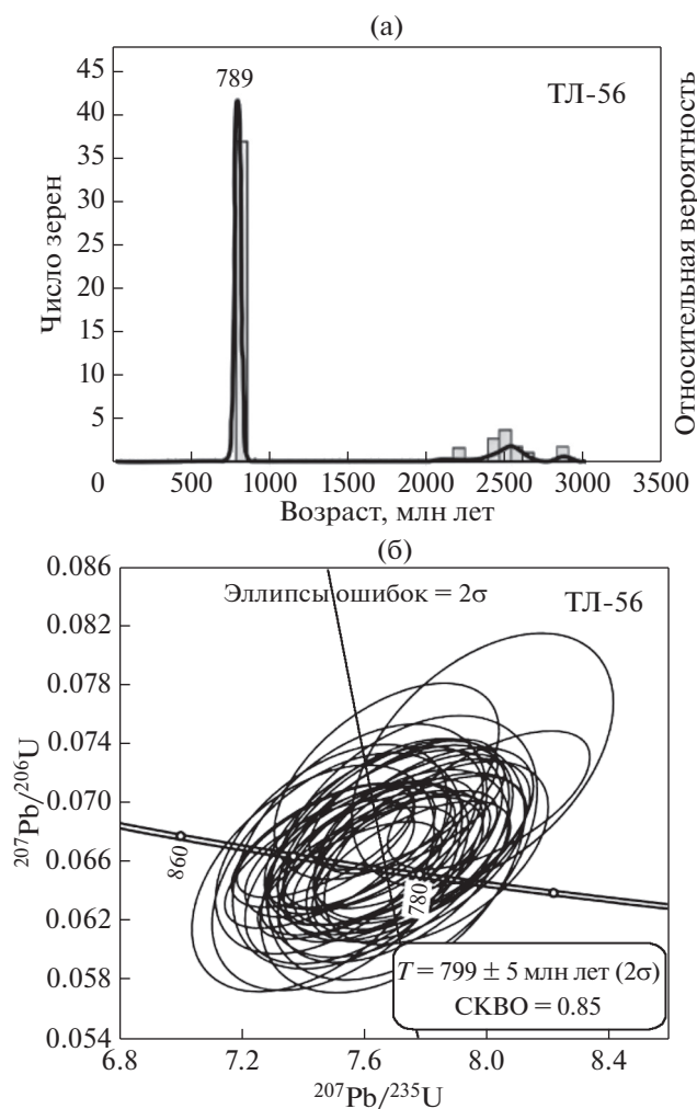
Рис. 10. Гистограмма и кривая относительной вероятности U-Pb возрастов (а) и диаграмма с конкордией (б) и для цирконов из туфитов (ТЛ-56) якшинской (тилимской) свиты.
