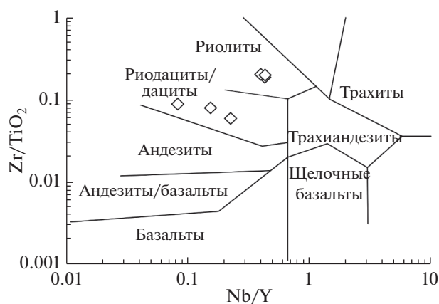
Рис. 4 Классификационная диаграмма Zr/TiO_2 - Nb/Y (Winchester, Flood, 1977) для кислых вулканитов якшинской свиты.
