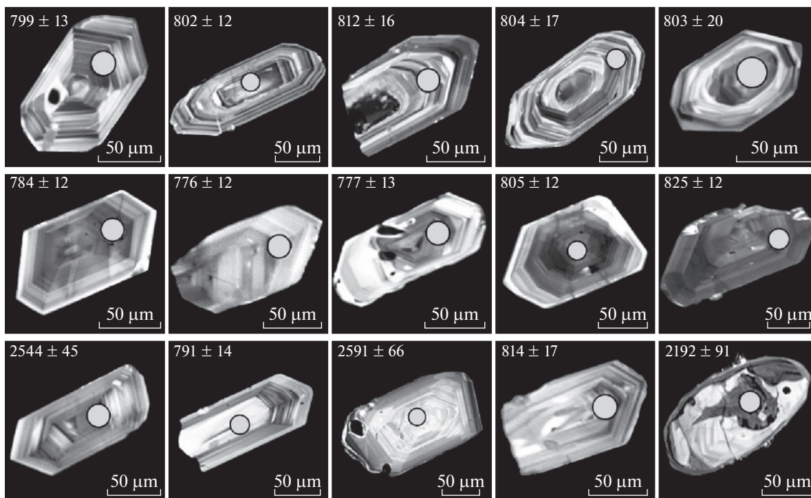
Рис. 8. Примеры кристаллов цирконов (катодоллюминесцентное фото) из кислых вулканитов якшинской (тилимской) и точерской свит. Первый ряд проба ТЛ-31, второй – ТЛ-39, третий – ТЛ-56.
