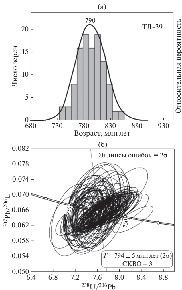
Рис. 11. Гистограмма и кривая относительной вероятности U-Pb возрастов (а) и диаграмма с конкордией (б) и для цирконов из риолита (ТЛ-39) точерской свиты.
