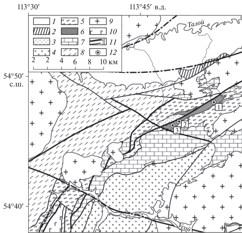
Рис. 2. Схематическая геологическая карта на основе геол. карты масштаба 1 : 200 000 (Гос. Геол. Карта, 2011). 1 – четвертичные отложения; 2 – имская свита ( K_{im} ); 3 – цаган-хунтейская свита ( T_{1ch} ); 4 – багдаринская свита ( D_3-C_2bg ); 5 – точерская свита ( D_3-C_1tc ); 6 – якшинская свита ( D_3jk ); 7 – ороченская свита ( D_{1-2or} ); 8 – сивоконская свита ( RF_3sk ); 9 – позднепалеозойские гранитоиды (витимканский комплекс); 10 – габбро-диориты шаманского комплекса ( RF_3 ); 11 – разломы (а – главные, б – второстепенные); 12 – Талойское месторождение марганца (показаны участки: 1 – Васильевский, 2 – Койдакон, 3 – Бугарикта).
