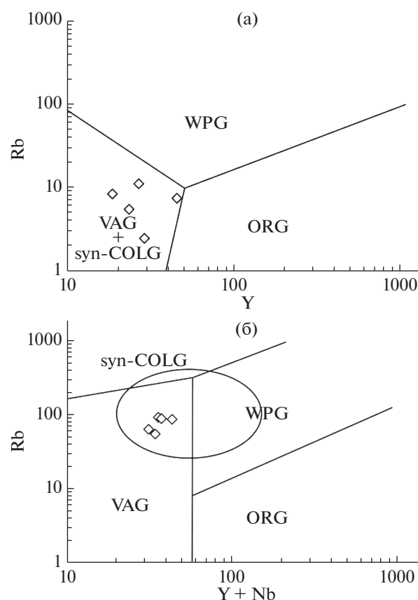
Рис. 7. Диаграмма Nb-Y (a) и Rb-(Y + Nb) (б) (Pearce et al., 1984; Pearce, 1996) для кислых вулканитов якшинской (тилимской) свиты. WPG — внутриплитные граниты, ORG — граниты океанических хребтов, VAG — граниты вулканических дуг и активных континентальных окраин, syn-COLG — синколлизонные граниты
