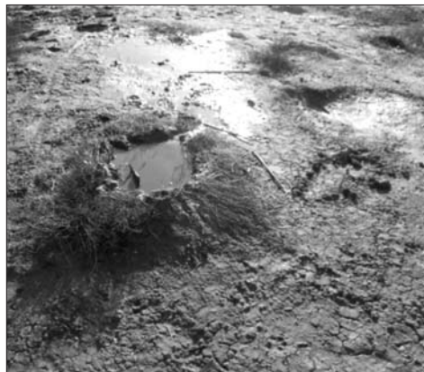
Рис. 9. Солдатско-Слободской грязевой вулкан. Активно газирующие сальзы вулкана
