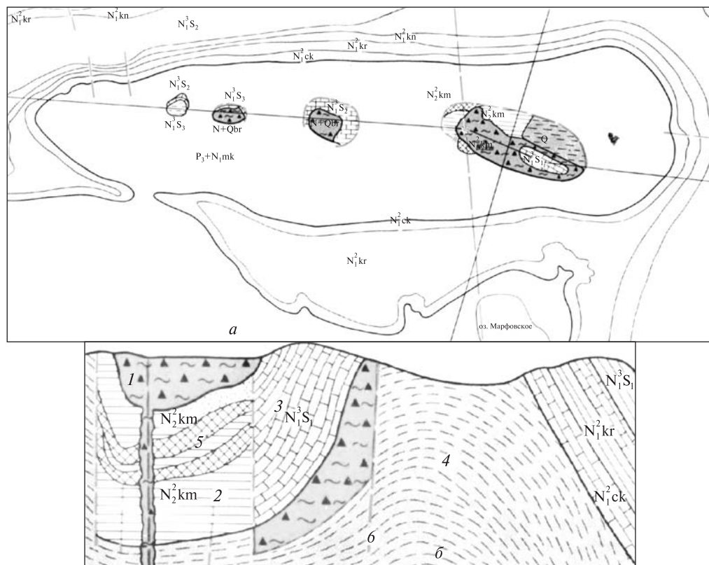
Рис. 4. Схема геологического строения Сартской антиклинали (а); разрез через Новоселовский грязевой вулкан (б): 1 — сопочная брекчия; 2 — вмещающая толща; 3 — известняки чокрака-сармата; 4 — глины майкопа; 5 — железные руды; 6 — разрывные нарушения
