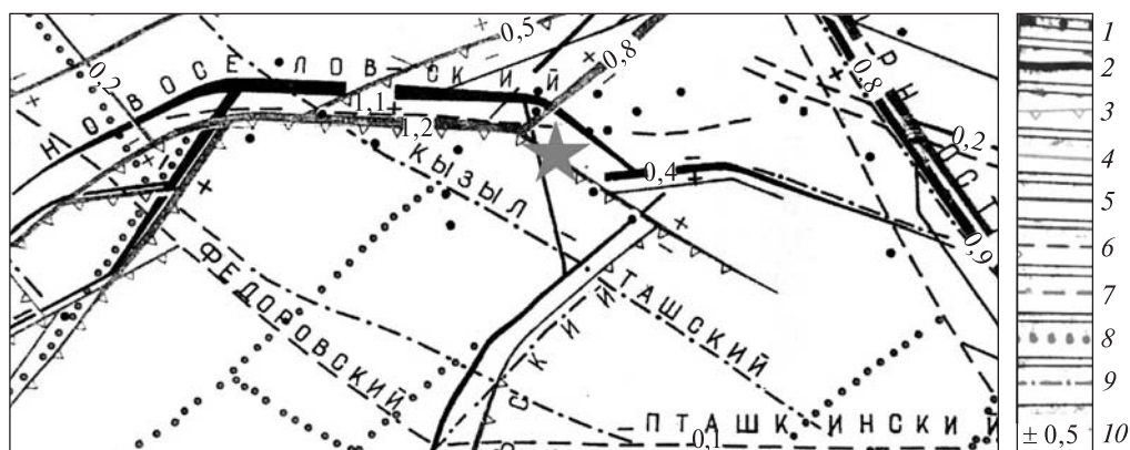
Рис. 5. Схема разрывных нарушений района Новоселовского грязевого вулкана. Разрывы, выраженные по поверхности: 1 — консолидированного фундамента; 2 — в отложениях юры (отражающий горизонт V); 3 — по подошве меловых отложений; 4 — по кровле нижнемеловых отложений; 5 — по подошве майкопских отложений; 6 — по кровле среднемайкопских отложений; 7 — по данным геологической съемки; 8 — по данным материалов аэрокосмической съемки; 9 — по данным геологической съемки и материалов аэрокосмической съемки; 10 — амплитуда разрывных нарушений по данным сейсморазведки электроразведки (в километрах). Толщина линий отражает амплитуду нарушений
