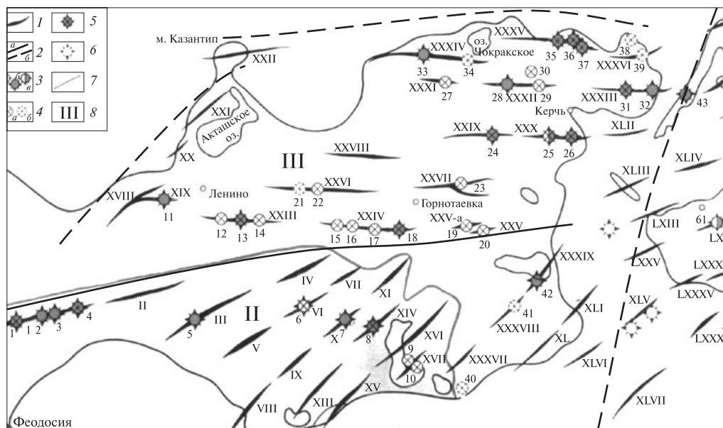
Рис. 1. Схема расположения грязевых вулканов Керченского полуострова: 1 — антиклинали; 2 — разрывные нарушения: а — достоверные, б — предполагаемые; 3 — грязевые вулканы (а — локбатанский тип, б — булганакский тип, в — шугинский тип); 4 — вдавленные синклинали (а — достоверные, б — предполагаемые); 5 — грязевые вулканы с вдавленными синклиналями; б — предполагаемые подводные грязевые вулканы; 7 — Парпачский гребень; 8 — Основные структурные элементы региона: II — мегантиклинорий Горного Крыма; III — южный борт Ингуло-Кубанского прогиба. Грязевые вулканы: 18 — Новоселовский, 25 — Джарджава, 26 — Солдатско-Слободской и Солнечный; XXIV — Сартская антиклиналь; XXX — Восходовская антиклиналь
