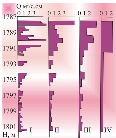
Рис. 5. Профили расхода для скважины 118. I – интервал усреднения 20 см. II – интервал усреднения 60 см. III – интервал усреднения 100 см. IV – усреднение по двум наиболее характерным интервалам кривой.
