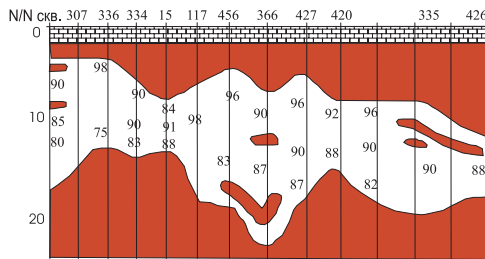
Рис.1. Профиль Бавлы, горизонт Д1. Цифрами на профилях обозначена нефтенасыщенность.
