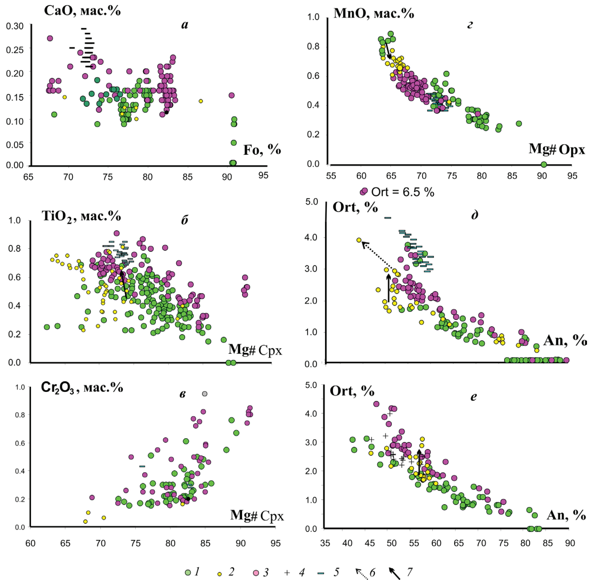
Рис. 5. Вариационные диаграммы составов минералов из пород массива Зиминых сопки: a–d — вкрапленники и субфенокристаллы из андезибазальтов: оливины ( a ), клинопироксены ( b , в ), ортопироксены ( г ), плагиоклазы ( д ); e — микролиты плагиоклаза. Минералы из пород ассоциаций: 1 — ассоциации I; 2 — ассоциации II; 3 — ассоциации III; 4 — из андезитов ассоциации III; 5 — из трахиандезибазальтов фундамента; 6 — тренд изменения состава плагиоклаза включение — минерал-хозяин; 7 — ортогональный тренд повышения калиевой щелочности пород.
