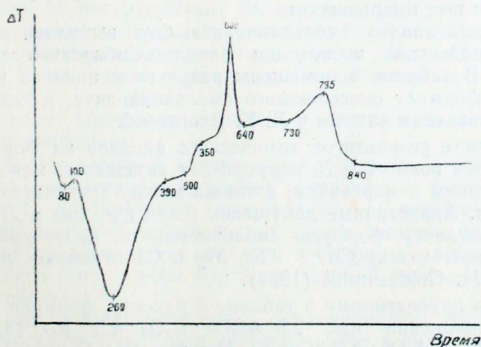
Рис. 3. Дифференциальная кривая нагревания смольяниновита.
