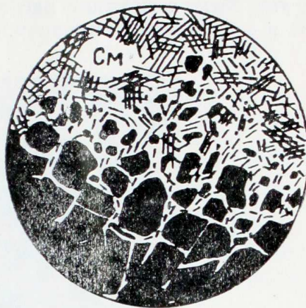
Рис. 1. Замещение кобальтина (черное) спутанноволокнистым агрегатом смоляниновита (См). Николи II. \times 160 .
