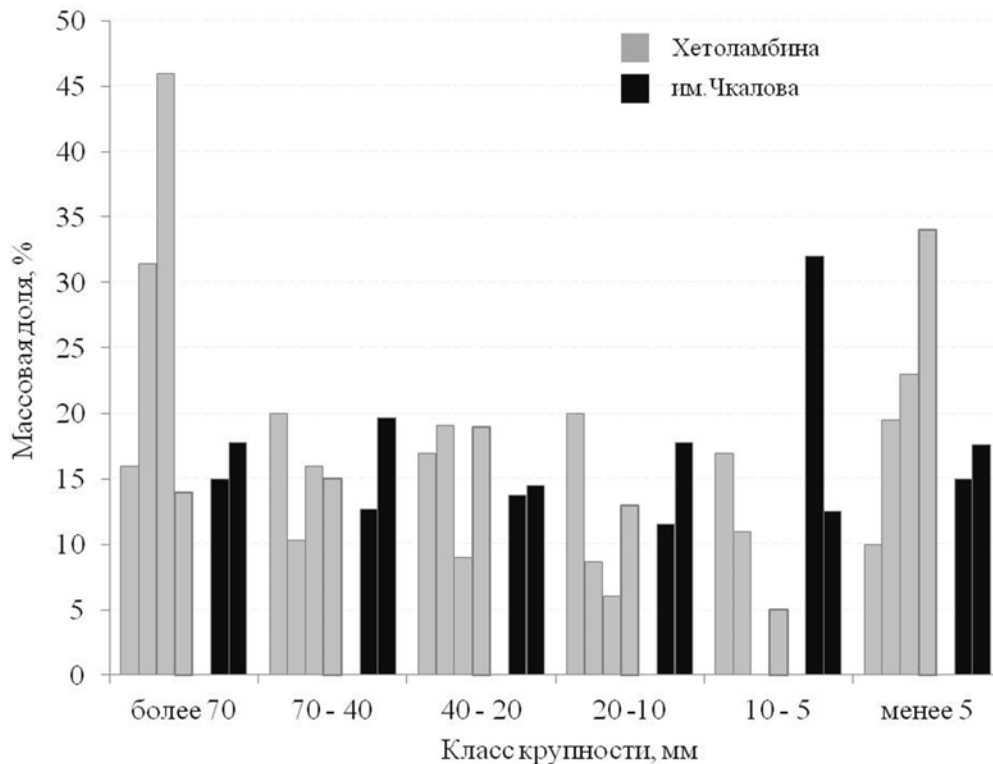
Рис. 4. Фракционный состав отвалов рудников Хетоламбина и им. Чкалова
