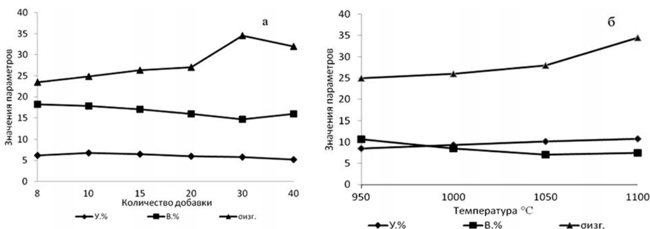
Рис. 7. Физико-механические свойства опытных изделий:
