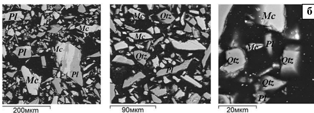
Рис. 6. Характеристика отходов обеспыливания ПОФ:
