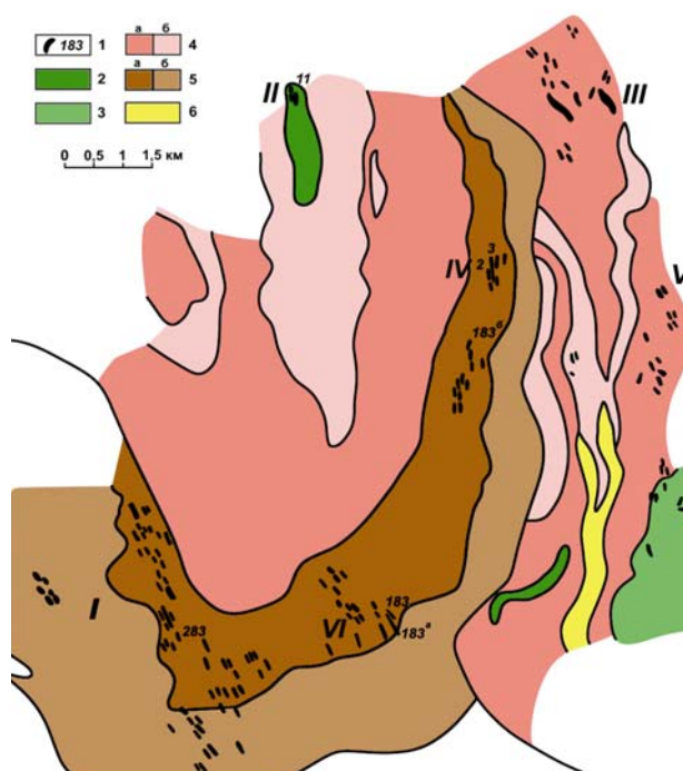
Рис. 1. Чупино-Лоухское пегматитовое поле: геологическая схематическая карта района Хетоламбинского месторождения [по: Чуйкина и др., 1971]:
