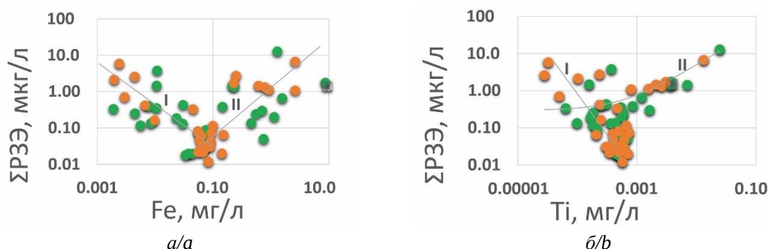
Рис. 5. Зависимость \Sigma P3Э от Fe (а) и Ti (б) в исследуемых подземных водах (усл. обознач. – на рис. 4) Fig. 5. Relationship between \Sigma REE and Fe (a) and Ti (b) in the studied groundwater (symbols are in Fig. 4)
