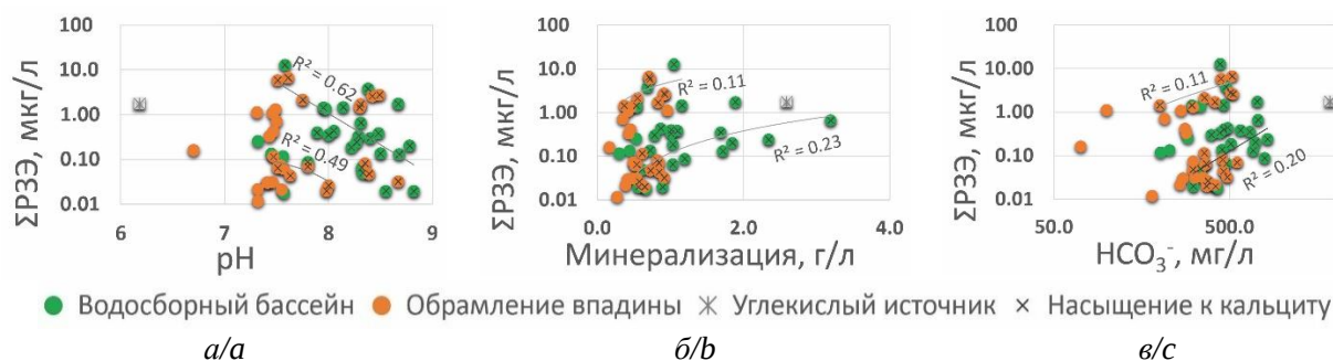
Рис. 4. Зависимость \Sigma P3Э от pH (а), общей минерализации (б) и HCO_3^- (в) в исследуемых подземных водах Fig. 4. Relationship between \Sigma REE and pH (a), TDS (b) and HCO_3^- (c) in the studied groundwater
