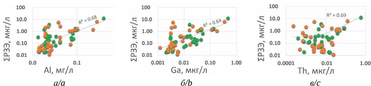
Рис. 6. Зависимость \Sigma P3Э от Al (а), Ga (б) и Th (в) в исследуемых подземных водах (усл. обознач. – на рис. 4) Fig. 6. Relationship between \Sigma REE and Al (a), Ga (b), Th (c) in the studied groundwater (symbols are in Fig. 4)
