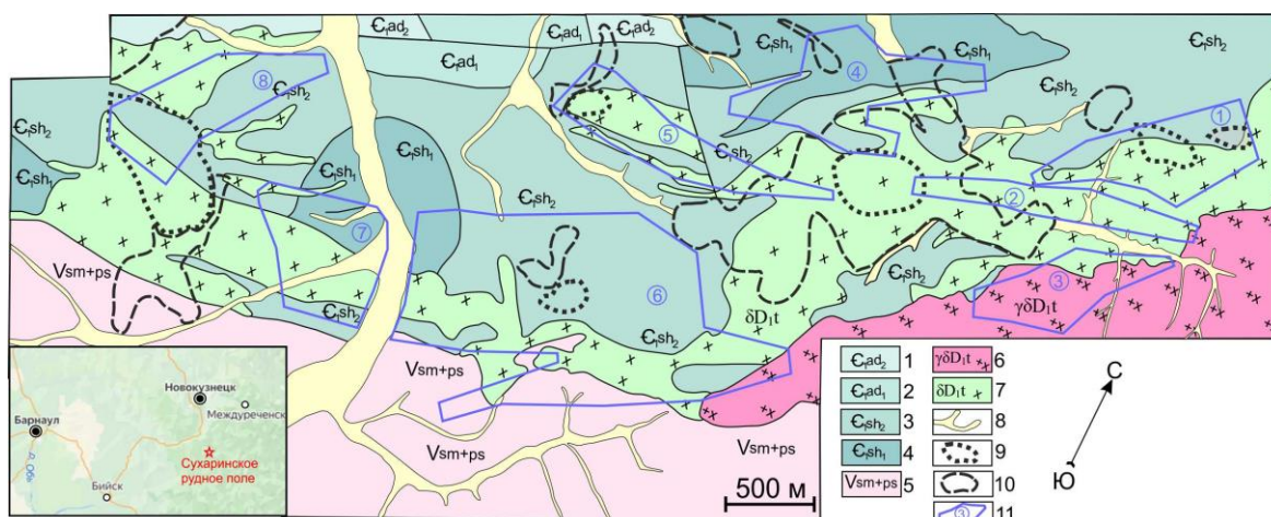
Рис. 1. Схема геологического строения Сухаринского рудного поля (по материалам ООО «Тетис-Т»): стратифицированные отложения: адиакая свита: 1 – верхняя подсвита ( \epsilon_{1ad2} ), известняки; 2 – нижняя подсвита ( \epsilon_{1ad1} ), известняки, алевролиты, конгломераты, базальты; сухаринская свита: 3 – верхняя пачка ( \epsilon_{1sh2} ), алевролиты, аргиллиты, известняки; 4 – нижняя пачка ( \epsilon_{1sh1} ), известняки, доломиты; 5 – объединенные самарская и пасекская толщи ( Vsm+ps ), метаморфические сланцы, алевролиты, известняки, вулканы основного и кислого состава; тельбесский магматический комплекс: 6 – гранодиориты; 7 – диориты; 8 – аллювиальные отложения; 9 – карьеры для добычи магнетитовой руды; 10 – отвалы карьеров; 11 – участки с выявленной золоторудной минерализацией: 1 – Аргыш-Таг, 2 – Дегтярный, 3 – Малиновы, 4 – Сухаринка Левобережная, 5 – Сухаринка Западная, 6 – Романовско-Кедровский, 7 – Самарский I-II, 8 – Самарский V
