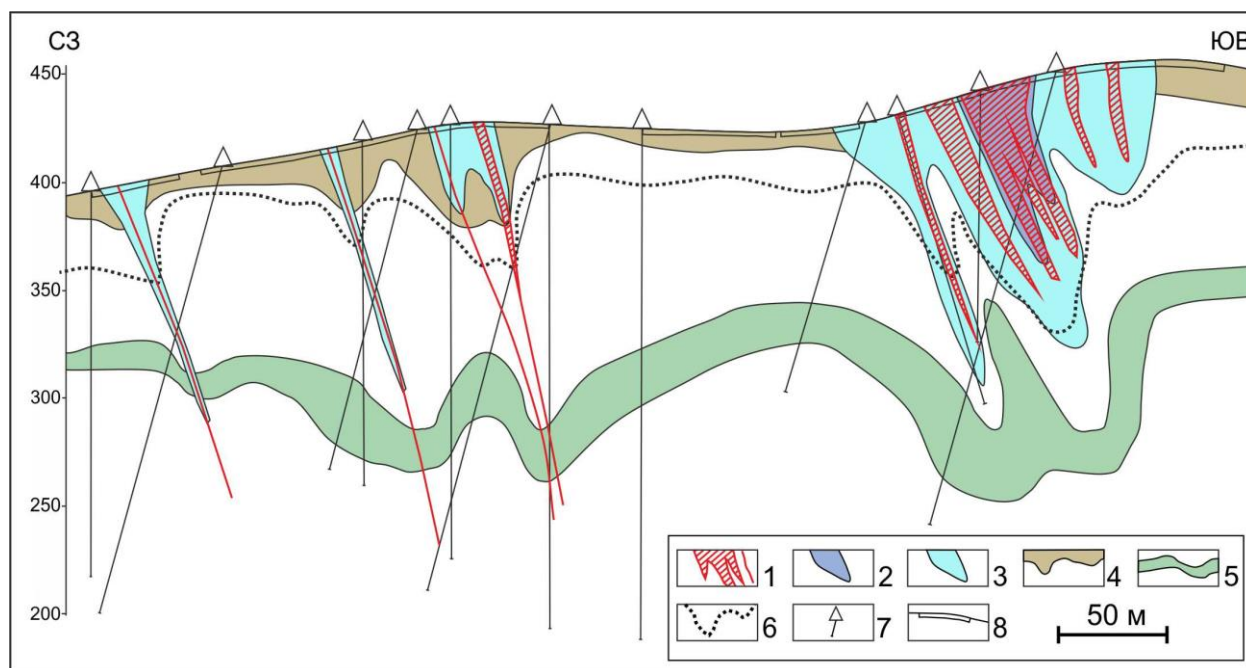
Рис. 6. Аномальные концентрации некоторых элементов в профиле площадной и линейных кор выветривания: 1 – Au > 1,0 г/т; 2 – Pb > 20 \cdot 10^{-3} %; 3 – Cu > 20 \cdot 10^{-3} %; 4 – участки развития геохимической ассоциации Ti, Ni, V, Zr (значения фактора 2 > 0,5 ); 5 – аномальные концентрации Sr ( > 40 \cdot 10^{-3} %); 6 – нижняя граница глинистой коры выветривания (зоны гидратации-начального гидролиза); 7 – буровые скважины; 8 – канавы и траншеи
