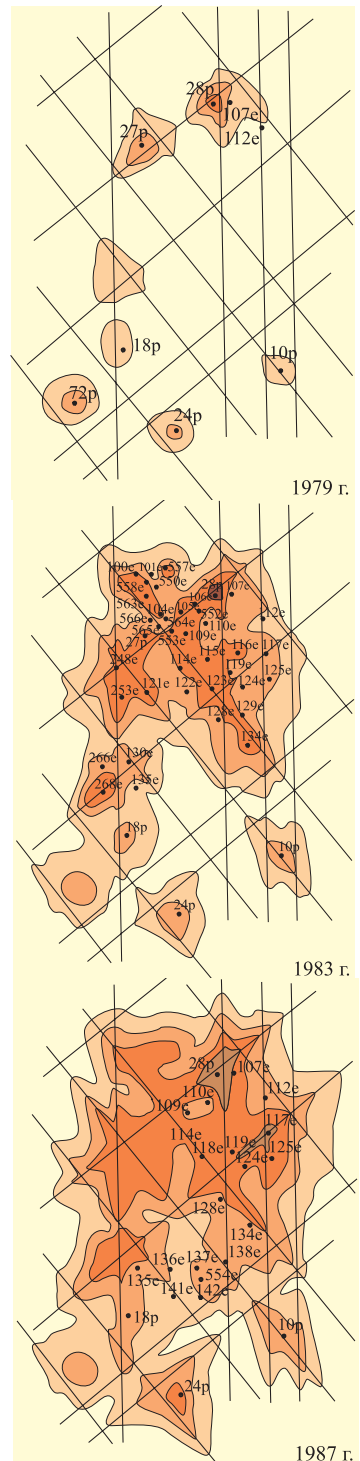
Рис. 3. Схема распределения пластового давления Лемниского участка 1979, 1983, 1987 гг.
