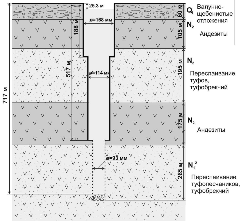
Рис. 1.4 – Строение скважины 1303 и геологический разрез.
