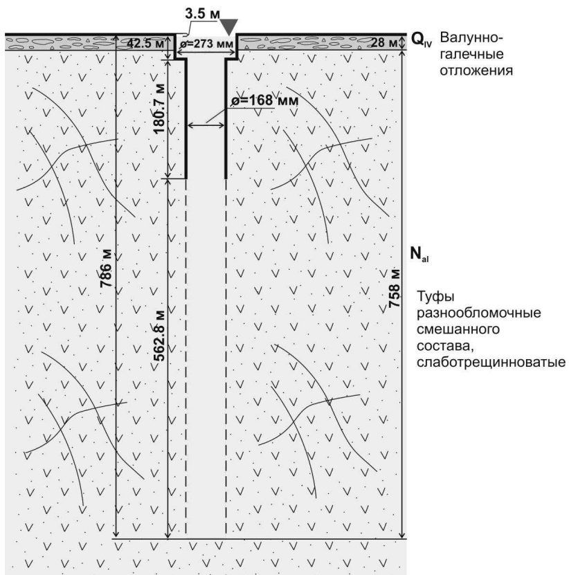
Рис. 1.5 – Строение скважины 1309 и геологический разрез.
