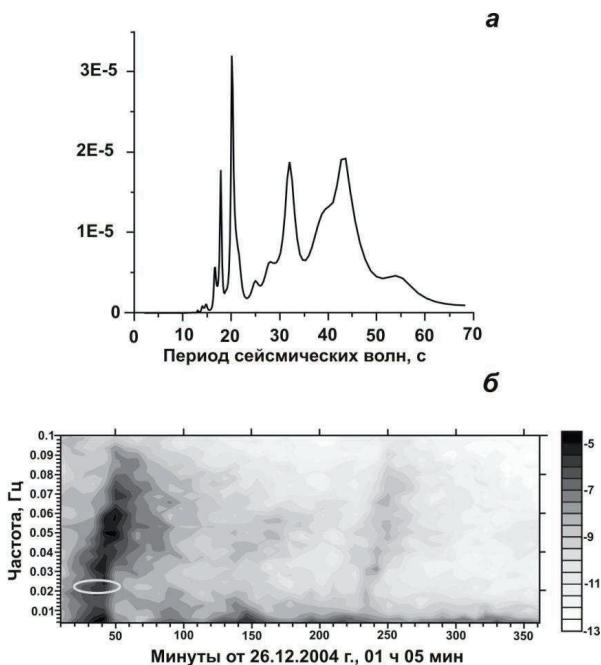
Рис. 3.2 – Спектры мощности смещений по каналу LHZ во время Суматра-Андаманского землетрясения 26.12.2004 г., сейсмостанция Петропавловск: а – спектр мощности по методу максимальной энтропии Бурга; б – динамический спектр, построенный в окне 10 минут с шагом 2 минуты. Эллипсом выделен частотный диапазон, соответствующий периодам поверхностных сейсмических волн 40-50 с.
