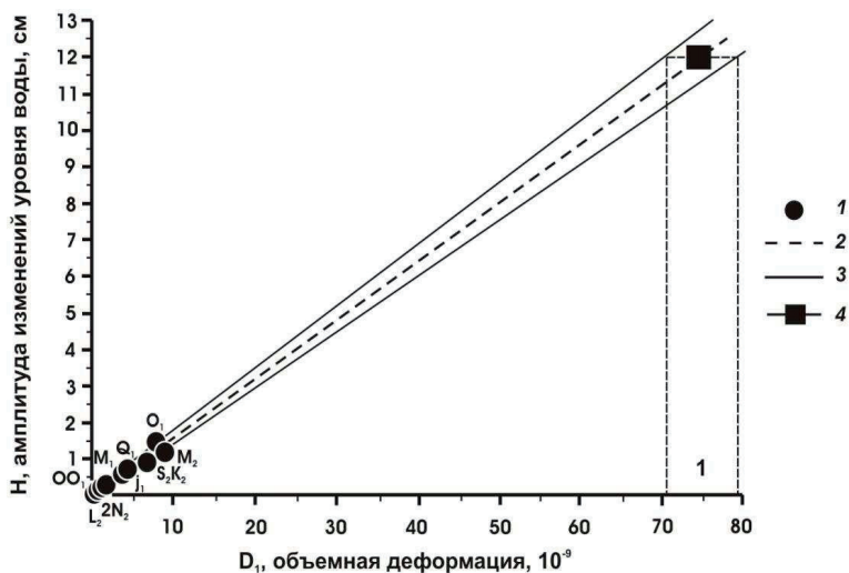
Рис. 3.9 – Зависимость выделенных приливных амплитуд в изменениях уровня воды H от теоретических величин приливной объемной деформации D_1 (табл. 3.1) для Кроноцкого землетрясения № 1 (табл. 3.2): 1 – приливные волны; 2 – тренд линейной зависимости амплитуд приливных волн в изменениях уровня воды от соответствующих величин приливной объемной деформации при значении коэффициента корреляции K=0.98 ; 3 – 95% доверительный интервал для линейной зависимости выделенных приливных амплитуд в изменениях уровня воды от величин теоретической приливной деформации; 4 – амплитуды косейсмических скачков во время землетрясений и диапазоны оценок косейсмической деформации.
