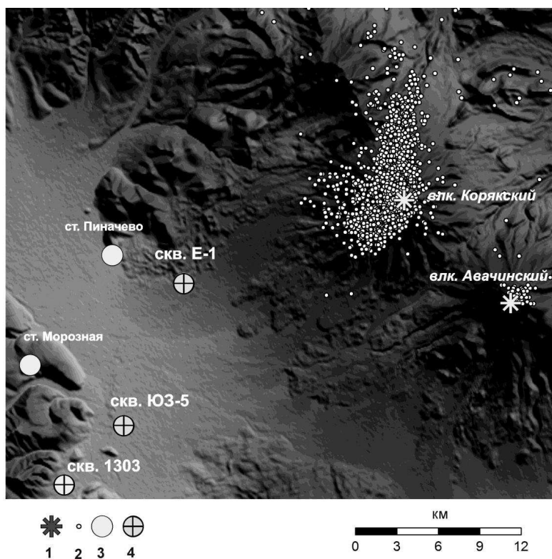
Рис. 4.2 – Карта района Авачинской вулканотектонической депрессии и ее обрамления. 1 – действующие вулканы; 2 – эпицентры роя землетрясений в районе вулкана Корякский 2008-2010 гг., K_S=3.1-8.3 ; 3 – пункты наблюдений за химическим составом подземных вод; 4 – наблюдательные пьезометрические скважины.
