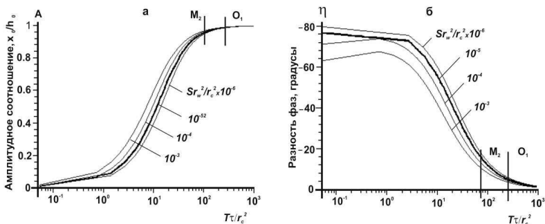
Рис. 2.8 – Графики изменений сдвига при различных значениях T/r_c^2 и Sr_w^2/r_c^2 для скважины 1303: а – амплитудное соотношение между изменениями уровня воды в скважине и гидростатического напора; б – фазовое запаздывание.
