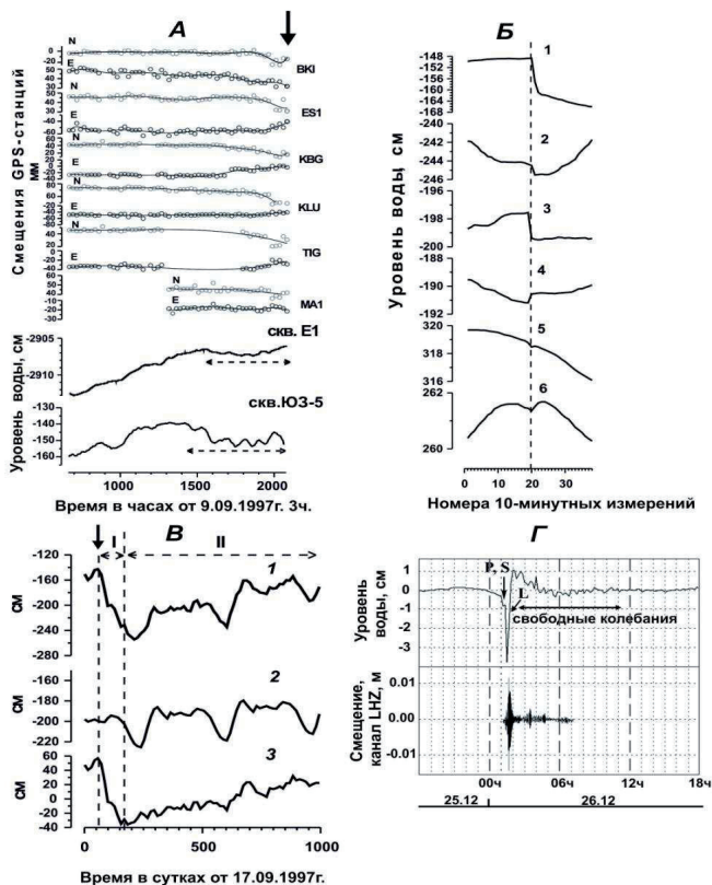
Рис. 1.11 – Типы вариаций уровня воды в скв. ЮЗ-5 под влиянием различных механизмов сейсмического воздействия: A – тип I – гидрогеодинамический предвестник Кроноцкого землетрясения: показан пунктирной линией; приводится в сопоставлении с перемещениями GPS-станций [Gordeev et al., 2001] и вариациями уровня воды в скважине E-1; B – тип II – косейсмические скачки уровня воды; B – тип III – понижение уровня воды после Кроноцкого землетрясения в течение 3.5 мес. (I) и его последующее восстановление в течение двух лет (II): 1 – данные наблюдений; 2 – выделенные годовая сезонность и линейный тренд, 3 – остатки в изменениях уровня воды после компенсации годовой сезонности и тренда; Г – тип IV – вынужденные и свободные колебания уровня воды в результате Суматра-Андаманского землетрясения приводятся в сопоставлении с записью смещений на канале LHZ, сейсмостанция Петропавловск.
