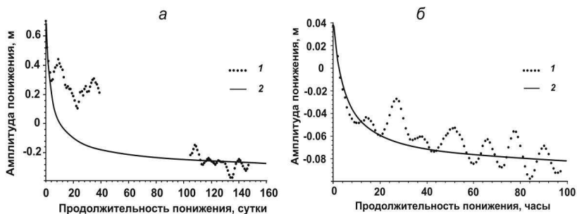
Рис. 3.6 – Результаты моделирования понижения уровня воды в скважинах (а) ЮЗ-5 после Кроноцкого землетрясения 5.12.1997 г. и (б) 1309 после Олюторского землетрясения 20.04.2006 г.: 1 – экспериментальные данные понижения уровня воды; 2 – теоретическое понижение уровня воды.
