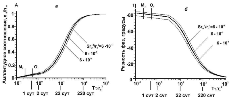
Рис. 4.4 – Характеристика инерционного эффекта водообмена в системе «скважина Е-1 – водовмещающая порода» с газом (а – амплитудное соотношение между изменениями уровня воды в скважине x_0 и напора h_0 ; б – фазовое запаздывание) в зависимости от периода вариаций \tau при различных значениях безразмерного параметра Sr_w^2/r_c^2 . M_2 , O_2 – приливные волны с периодами 12.42 ч и 25.82 ч соответственно. Жирными линиями показаны наиболее вероятные приближения модели к фактическим данным. По горизонтальным осям вертикальными линиями отмечены значения периода вариаций \tau .
