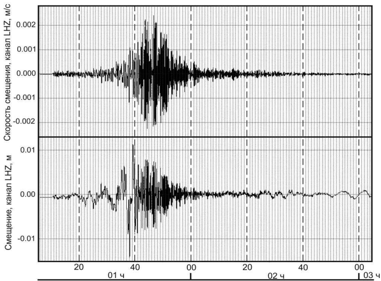
Рис. 3.1 – Запись Суматра-Андаманского землетрясения от 26.12.2004 на канале LHZ на сеймостанции Петропавловск. Сейсмические волны регистрировались более 50 минут: с 1 часа 10 минут до примерно двух часов.
