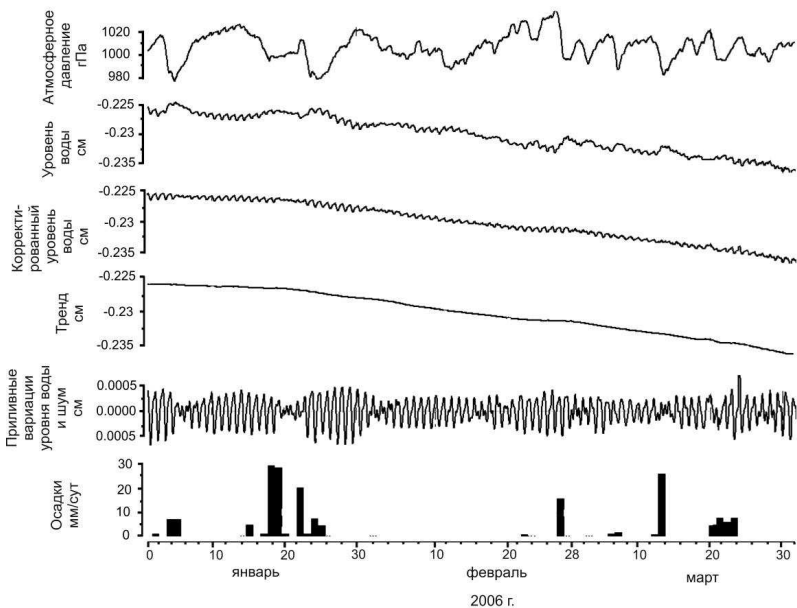
Рис. 1.8 – Среднечасовые данные наблюдений за атмосферным давлением и уровнем воды, скважина 1303, 1.01.2006 г.-1.04.2006 г., в сопоставлении с суточными осадками. Представлены также изменения уровня воды с компенсированными баровариациями, выделенные тренд и высокочастотная составляющая в изменениях уровня воды.
