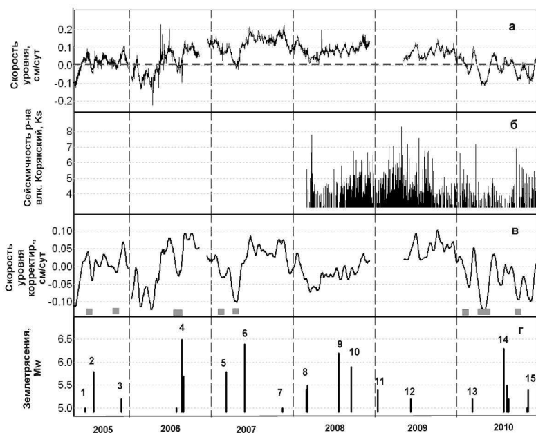
Рис. 1.15 – Вариации уровня воды скважине Е-1 в 2005-2010 гг. в сопоставлении с развитием сейсмичности в районе вулкана Корякский и сильными землетрясениями: а – суточная скорость изменения уровня воды с компенсированными баровариациями (жирной линией показано осреднение среднесуточных данных в окне 15 сут); б – землетрясения в районе вулкана Корякский с K_S \geq 4.0 ; в – среднесуточная скорость изменения уровня воды, скорректированная за счет средней скорости тренда в течение соответствующего фрагмента (горизонтальными линиями обозначены времена проявления гидрогеодинамического предвестника); г – землетрясения с M_w \geq 5.0 на расстоянии R \leq 350 км от скважины; цифрами обозначенным номера сейсмических событий в соответствии с табл. 1.4.
