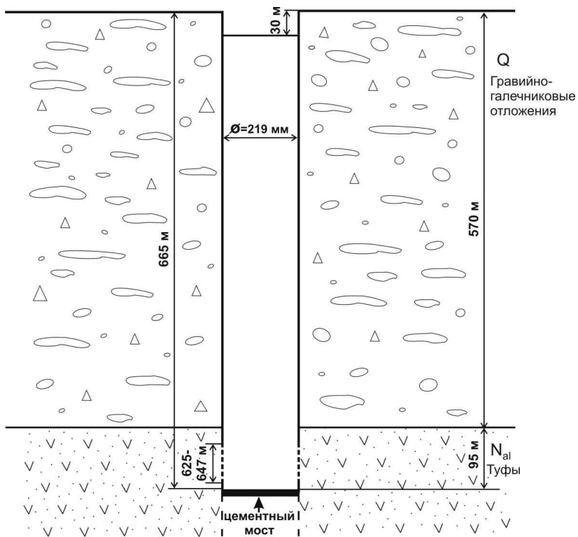
Рис. 1.3 – Строение скважины Е-1 и геологический разрез.
