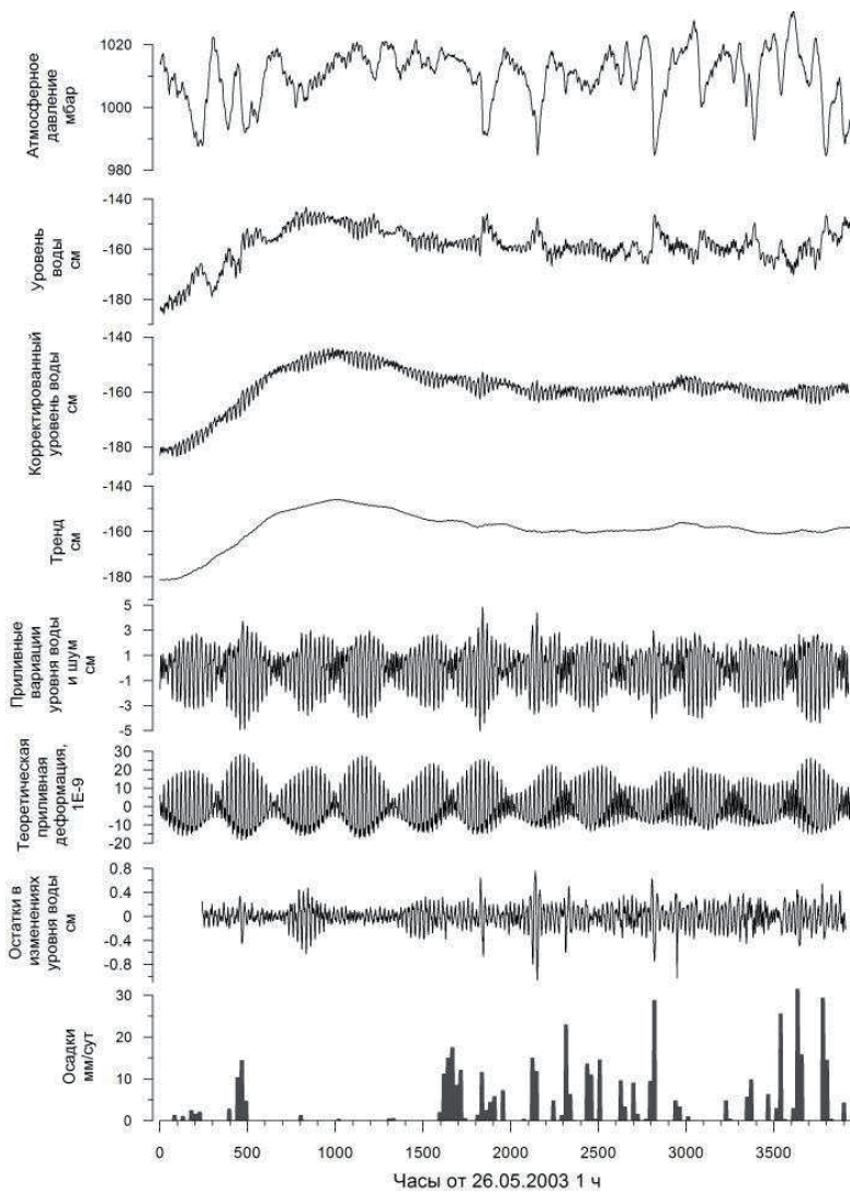
Рис. 1.6 – Среднечасовые данные наблюдений за атмосферным давлением и уровнем воды, скважина ЮЗ-5, 26.05.2003 г.-5.11.2003 г., в сопоставлении с суточными осадками. Представлены также изменения уровня воды с компенсированными баровариациями, выделенные тренд и высокочастотная составляющая в изменениях уровня воды, остаточные изменения уровня после компенсации барометрических и приливных вариаций.
