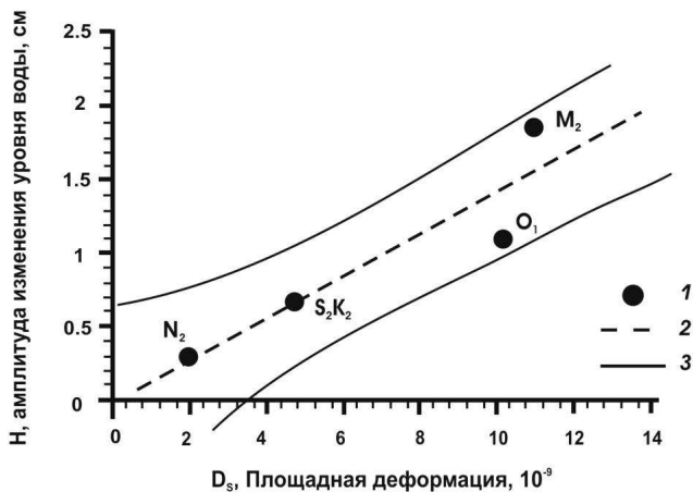
Рис. 2.4 – Характеристика приливного отклика уровня воды в скважине 1303: 1 – зависимость выделенных приливных амплитуд в изменениях уровня воды от величин теоретической приливной деформации (табл. 2.26); 2 – тренд (линейная связь между этими величинами при значении коэффициента регрессии 0.85); 3 – 95% доверительный интервал для зависимости выделенных приливных амплитуд в изменениях уровня воды от величин теоретической приливной деформации.
