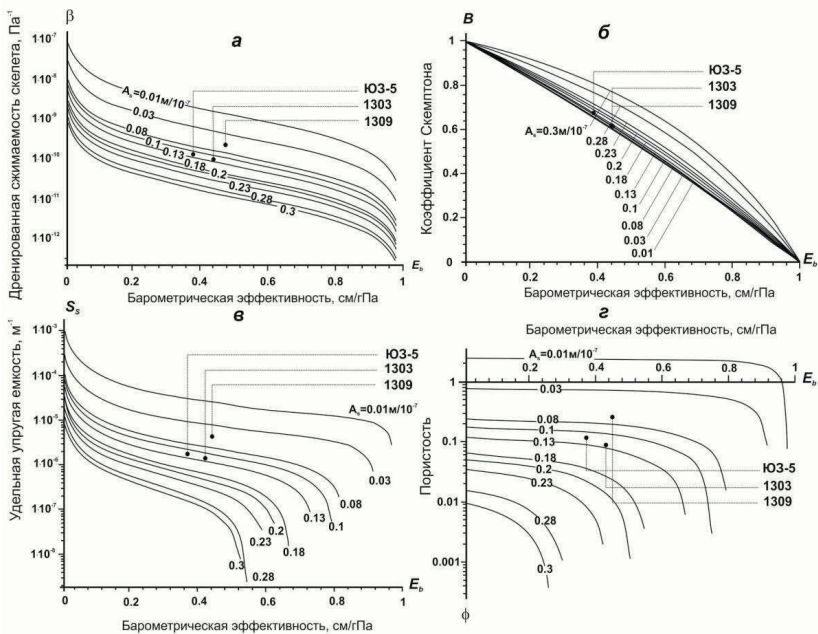
Рис. 2.6 – Связь упругих параметров водовмещающих пород, вскрытых пьезометрической скважиной: a – сжимаемости скелета водовмещающей породы \beta по (1.19), б – коэффициента Скемптона B по (1.20), в – удельной упругой емкости S_s по (1.22), г – пористости водовмещающих пород \phi по (1.23), и величин барометрической эффективности E_b и приливной чувствительности уровня воды A_s для статически изолированных условий в системе «скважина – водовмещающая порода».
