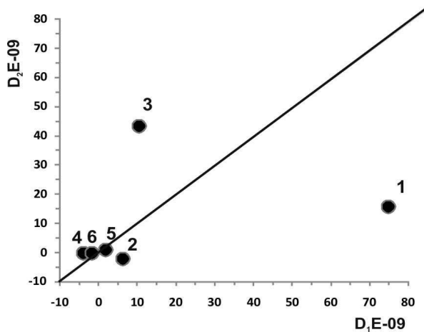
Рис. 3.12 – Соотношение величин косейсмической объемной деформации, полученных по данным урвнемерных наблюдений D_1 и по модели дислокационного источника D_2 . Номера соответствуют номерам землетрясений по табл. 3.2.
