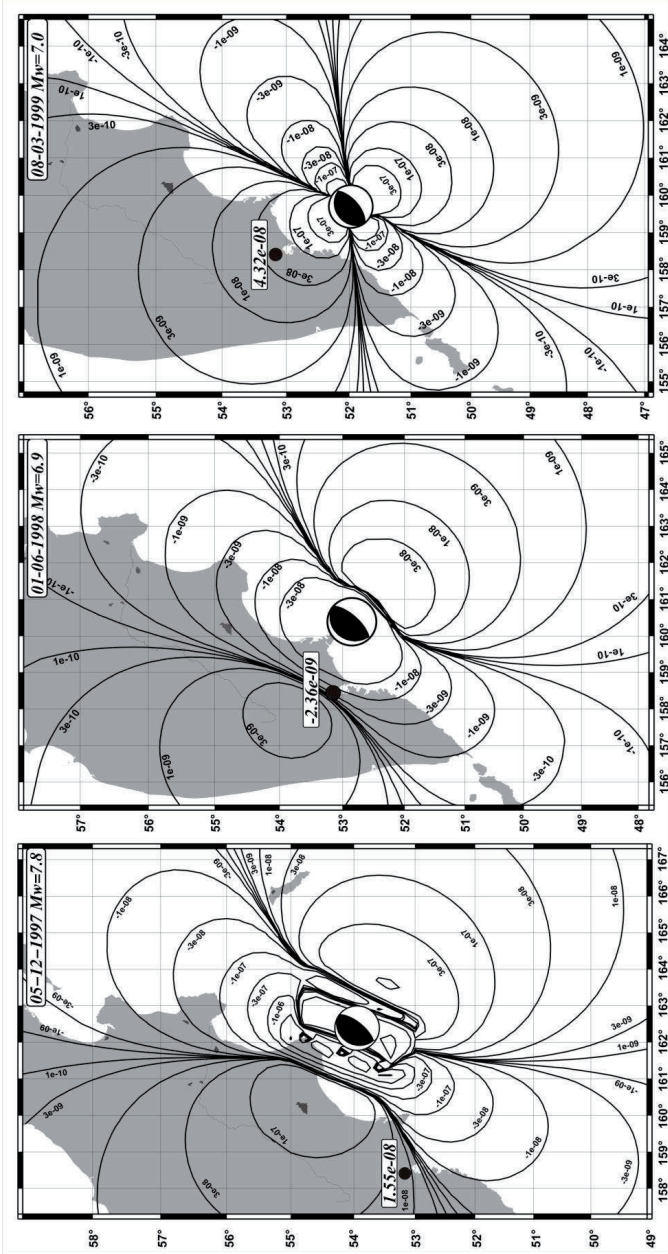
Рис. 3.10 – Горизонтальное распределение объемной косейсмической деформации на глубине 500 м по модели дислокационного источника для землетрясений № 1-3 (табл. 3.2) с указанием величин деформации в районе скважины ЮЗ-5 (показана черным кружком) [Копылова, Стеблов, Болдина и др., 2010].
