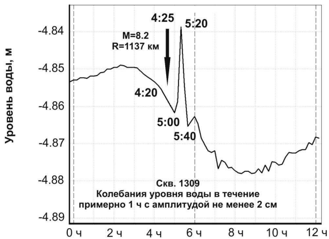
Рис. 1.14 – Вариации уровня воды в скважинах 1303, 1309 в связи с землетрясением Симуширское-2 13.01.2007 г. (по данным 10-минутной регистрации).
