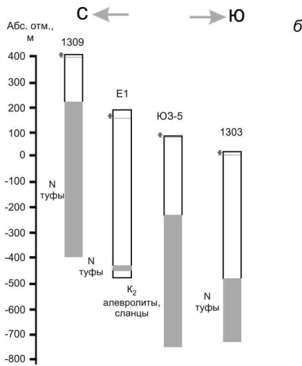
Рис. 1.1 – Схемы расположения наблюдательных скважин (а) и их строения (б): 1 – скважины ОАО «Камчатгеология»; 2 – скважины КФ ГС РАН.
