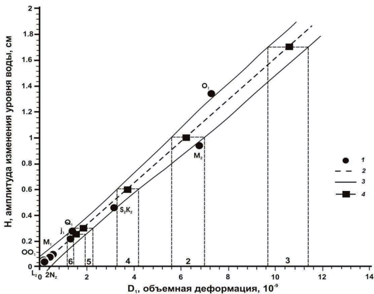
Рис. 3.8 – Зависимость выделенных приливных амплитуд в изменениях уровня воды H от теоретических величин приливной объемной деформации D_1 (табл. 3.1) для землетрясений № 2-6 (табл. 3.2): 1 – приливные волны; 2 – тренд линейной зависимости амплитуд приливных волн в изменениях уровня воды от соответствующих величин приливной объемной деформации при значении коэффициента корреляции K=0.98 ; 3 – 95% доверительный интервал для линейной зависимости выделенных приливных амплитуд в изменениях уровня воды от величин теоретической объемной приливной деформации; 4 – амплитуды косейсмических скачков во время землетрясений и диапазоны оценок косейсмической деформации.
