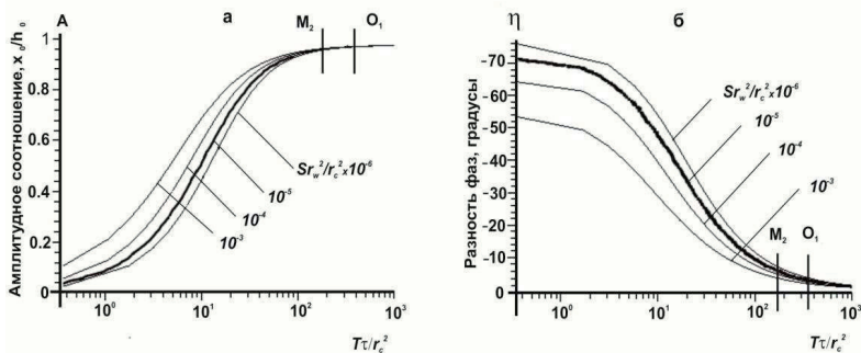
Рис. 2.9 – Графики изменений сдвига при различных значениях T/r_c^2 и Sr_w^2/r_c^2 для скважины 1309: а – амплитудное соотношение между изменениями уровня воды в скважине и гидростатического напора; б – фазовое запаздывание.
