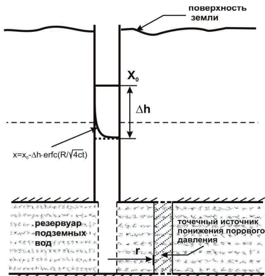
Рис. 1.20 – Схема формирования постсейсмического понижения уровня воды в скважине, вскрывающей изолированные водовмещающие породы: x_0 – начальный уровень воды в скважине, \Delta h = \Delta p / \rho g – изменение гидростатического напора при изменении порового давления \Delta p , где \Delta p – амплитуда понижения порового давления; x – изменение уровня воды, R – радиус чувствительности скважины к источнику падения порового давления в водовмещающих породах.
