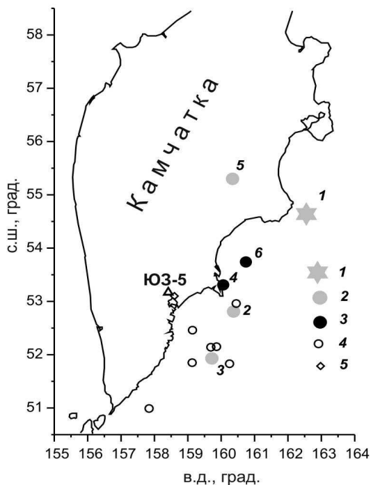
Рис. 1.10 – Схема расположения скважины ЮЗ-5 и эпицентров землетрясений: 1 – Кроноцкое землетрясение 5.12.1997 г., M_w=7.8 ; 2 – землетрясения, вызвавшие косейсмическое понижение уровня воды; 3 – землетрясения, вызвавшие косейсмическое повышение уровня воды (номера землетрясений соответствуют номерам в таблице 1.3 и на рис. 1.11); 4 – землетрясения с M_w=5.3-5.9 на гипоцентральной дистанции от скважины R=100-250 км, произошедшие в периоды детальных наблюдений (табл. 1.2) и не вызвавшие изменения уровня воды (их относительное воздействие в районе скважины показано на рис. 1.11); 5 – метеостанция Пионерская.
