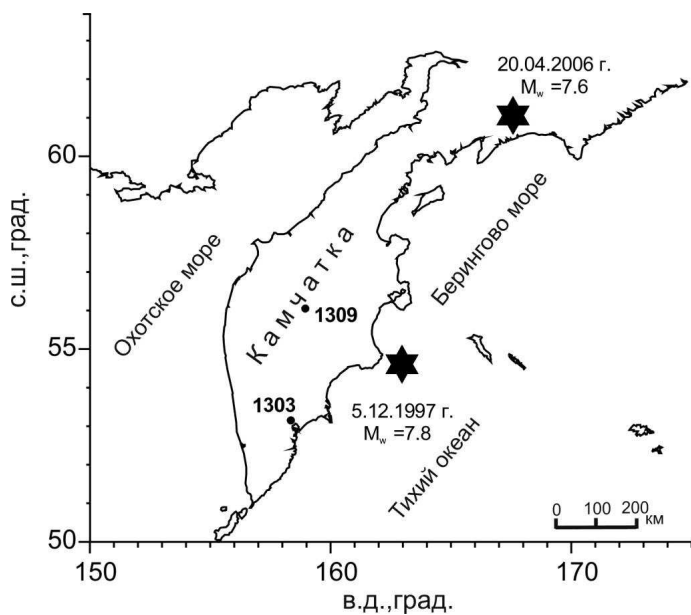
Рис. 1.12 – Схемы расположения скважин 1303 и 1309. Звездами показаны эпицентры землетрясений Кроноцкого 05.12.1997 г. и Олюторского 20.04.2006 г.
