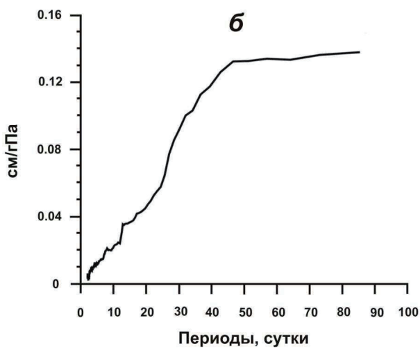
Рис. 2.2 – Амплитудные передаточные функции от вариаций атмосферного давления к изменениям уровня воды в скважине Е-1: а – в диапазоне часовых вариаций; б – в диапазоне суточных вариаций для скважины Е-1.
