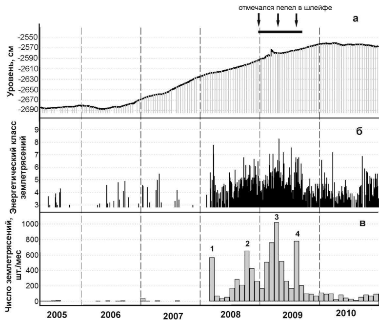
Рис. 1.16 – Изменение уровня воды в скважине Е-1 в 2005-2010 гг. в сопоставлении с развитием сейсмичности и парогозовой активности вулкана Корякский: а – изменения уровня воды по данным цифровых и ручных измерений (приводятся в глубинах уровня ниже оголовка скважины); горизонтальной линией показан интервал времени фреатического извержения; б – землетрясения с величинами энергетических классов K_5=3.1-8.3 в районе вулкана Корякский; в – суммарное за месяц количество землетрясений (цифрами обозначены максимумы сейсмической активности: 1 – март 2008 г., 2 – октябрь 2008 г., 3 – апрель 2009 г., 4 – август 2009 г.).
