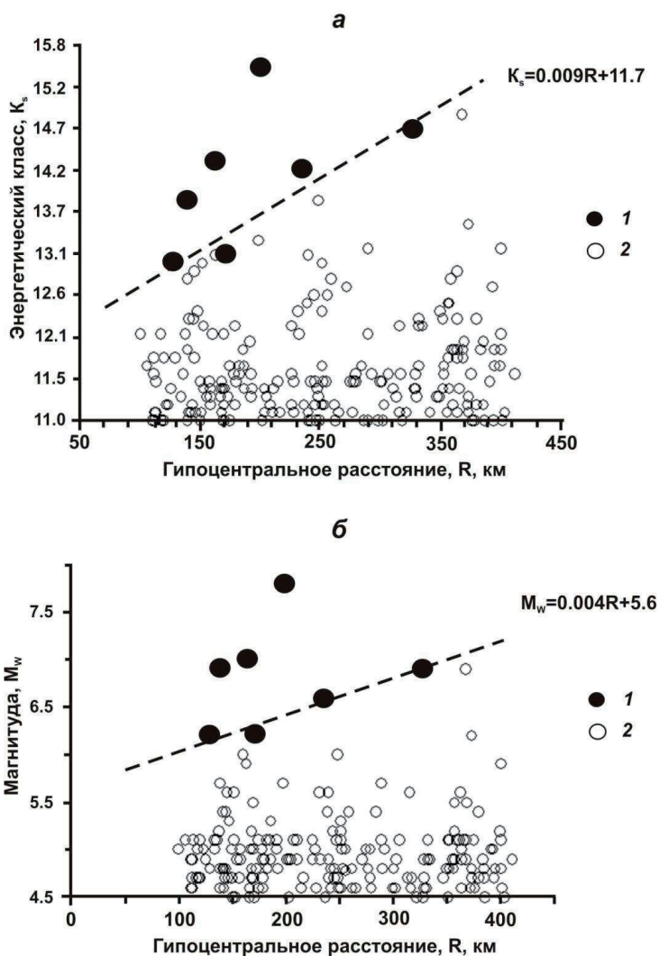
Рис. 3.13 – Зависимости проявления косейсмических скачков в вариациях уровня воды в скважине ЮЗ-5 от параметров землетрясений: энергетического класса K_s (а), магнитуды M_w (б) и гипоцентрального расстояния R , км: 1 – землетрясения, сопровождавшиеся косейсмическими скачками в изменении уровня воды в скважине ЮЗ-5; 2 – землетрясения, не сопровождавшиеся косейсмическими скачками в изменении уровня воды.
