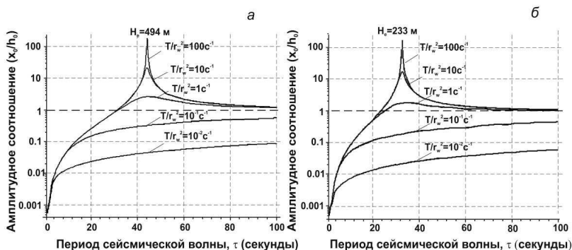
Рис. 3.3 – Изменение амплитудного соотношения между вариациями уровня воды в скважинах ЮЗ-5 (а), 1309 (б) и изменением напора x_0/h_0 в зависимости от параметра системы «скважина – водовмещающая порода» T/r_w^2 и периода сейсмической волны \tau .
