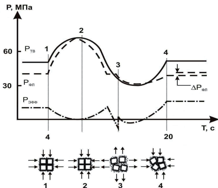
Рис. 3.5 – Изменение обжимающего ( P_{ТВ} ), порового ( P_{ФЛ} ) и эффективного ( P_{ЭФФ} ) давлений при прохождении сейсмической волны через горную породу [Шмонов и др., 2002]: 1 – исходное состояние системы вода-порода; 2 – фаза повышения обжимающего и порового давлений и сжатия образца; 3 – фаза падения давления обжима, разрушение образца под действием порового давления; 4 – фаза сжатия, механическая дилатансия образца; \Delta P_{ФЛ} – падение порового давления в результате нарушения структуры образца после сейсмической вибрации.
