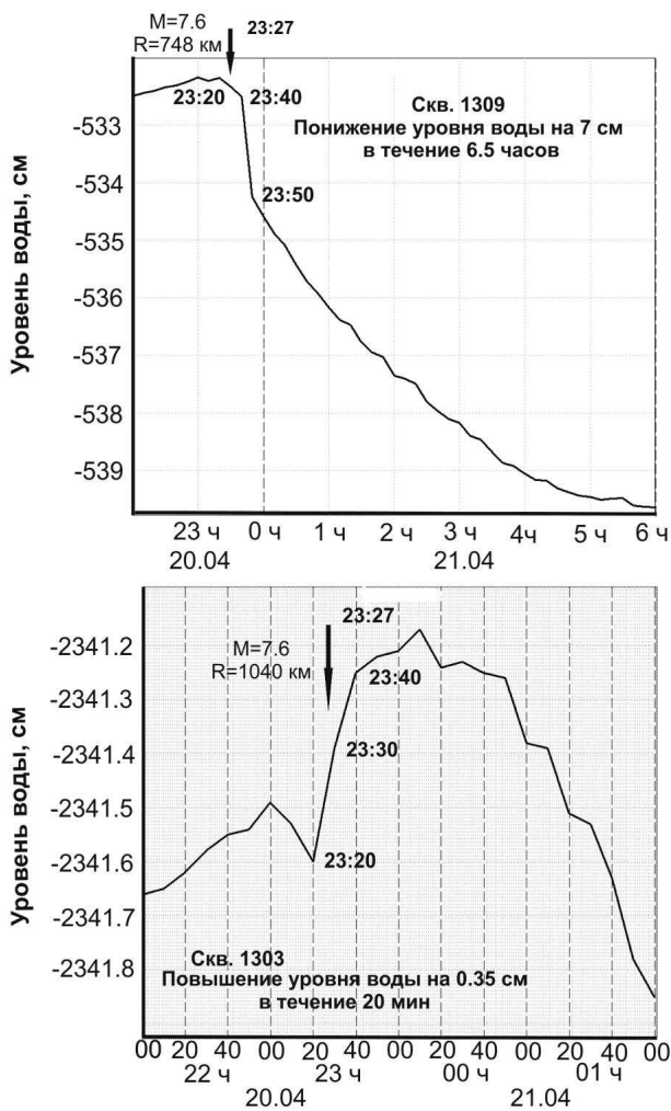
Рис. 1.13 – Вариации уровня воды в скважинах 1309, 1303 в связи с Олоторским землетрясением 20.04.2006 г. (по данным 10-минутной регистрации).
