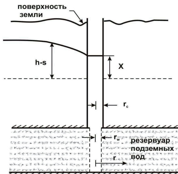
Рис. 1.18 – Схема формирования отклика уровня воды в скважине на гармонические вариации порового давления в изолированных водовмещающих породах при воздействии приливных волн: r – горизонтальное расстояние от центра скважины, r_w – радиус скважины в области ее связи с водовмещающими породами, r_c – радиус скважины в области, где происходят колебания уровня воды, h – изменение гидростатического напора, s – понижение напора (положительное направление вниз), X – изменение уровня воды.
