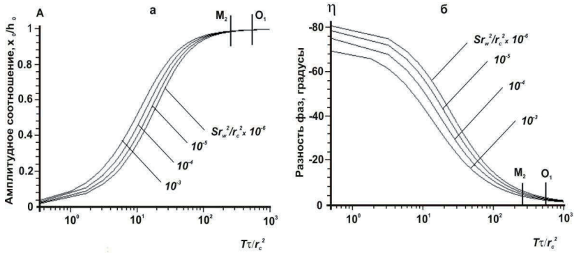
Рис. 2.7 – Графики изменений сдвига при различных значениях T/r_c^2 и Sr_w^2/r_c^2 для скважины ЮЗ-5: а – амплитудное соотношение между изменениями уровня воды в скважине и гидростатического напора; б – фазовое запаздывание.
