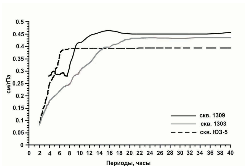
Рис. 2.1 – Амплитудные передаточные функции от вариаций атмосферного давления к изменениям уровня воды в скважинах ЮЗ-5, 1303 и 1309.
