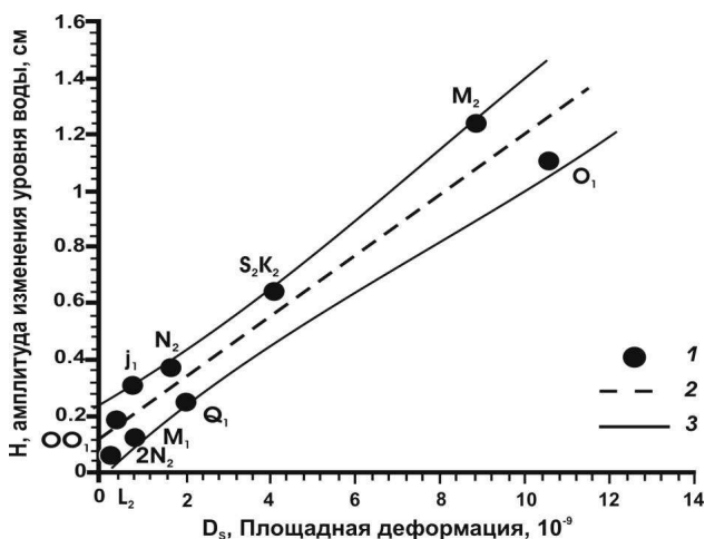
Рис. 2.5 – Характеристика приливного отклика уровня воды в скважине 1309: 1 – зависимость выделенных приливных амплитуд в изменениях уровня воды от величин теоретической приливной деформации (табл. 2.2в); 2 – тренд (линейная связь между этими величинами при значении коэффициента регрессии 0.93); 3 – 95% доверительный интервал для зависимости выделенных приливных амплитуд в изменениях уровня воды от величин теоретической приливной деформации
